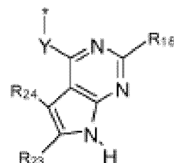
formule (IIIa-3)
