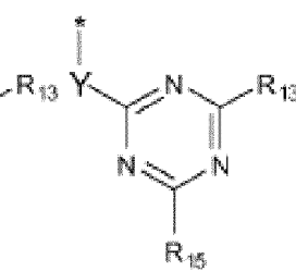
formule (IIb-3)
