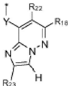
formule (IIIa-22)
