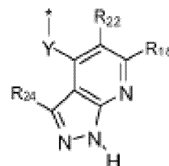
formule (IIIa-6)
