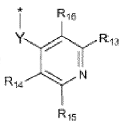
formule (IIb-1)
