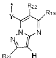
formule (IIIa-14)
