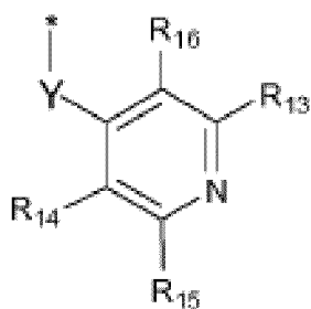
formule (IIb-1)
