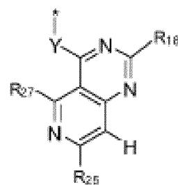
formule (IIIb-6)
