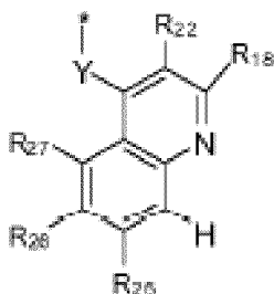
formule (IIIb-1)
