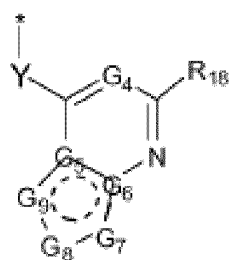
formule (IIIa)
