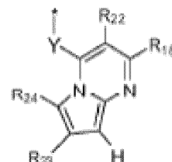
formule (IIIa-12)
