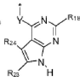
formule (IIIa-3)
