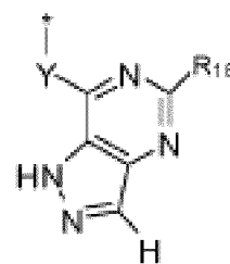
formule (IIIa-9)
