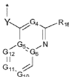
formule (IIIb)
