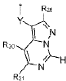
formule (IIId-2)
