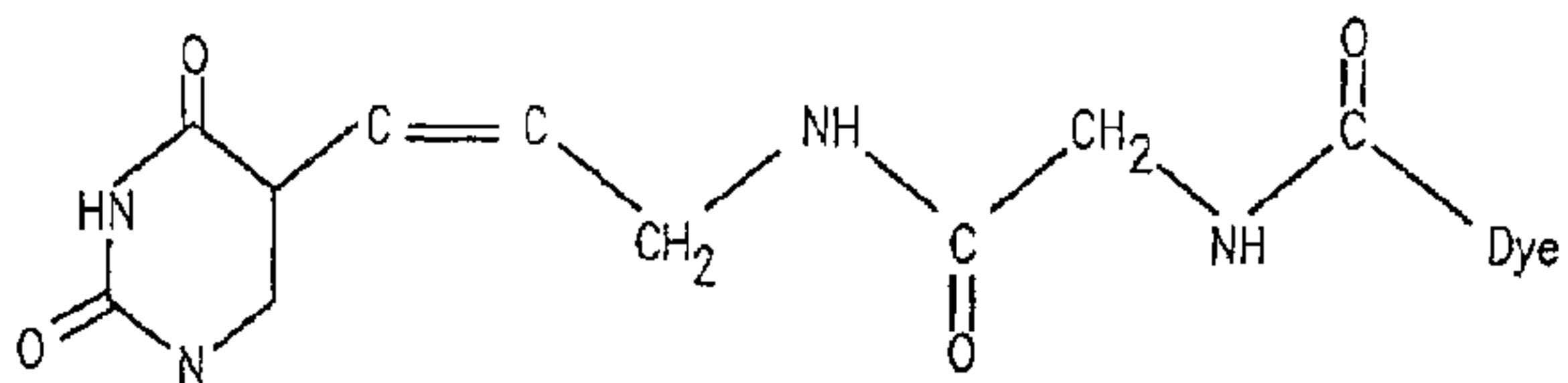
Diglycinyyl linker
