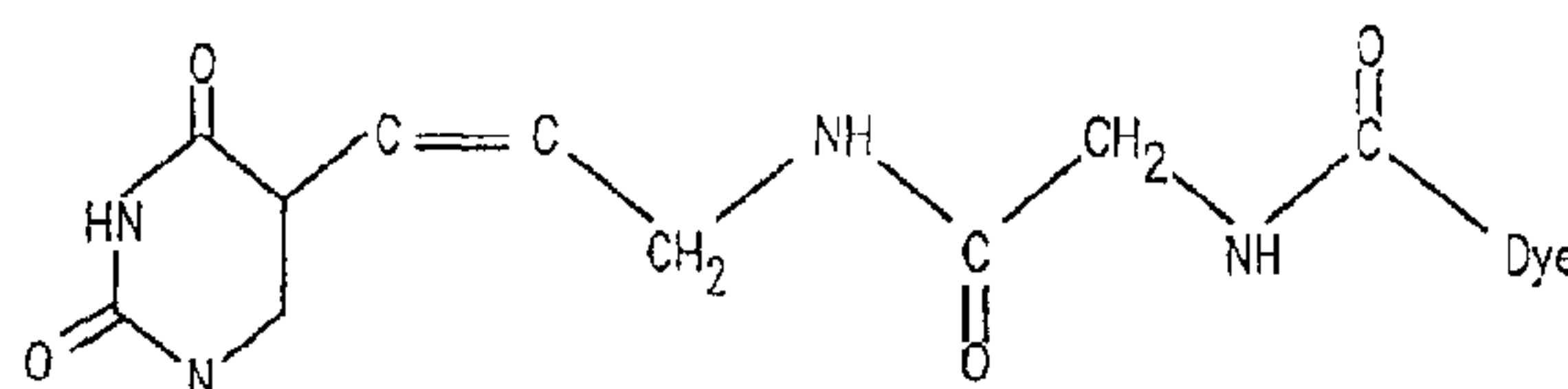
Diglycinyll linker
