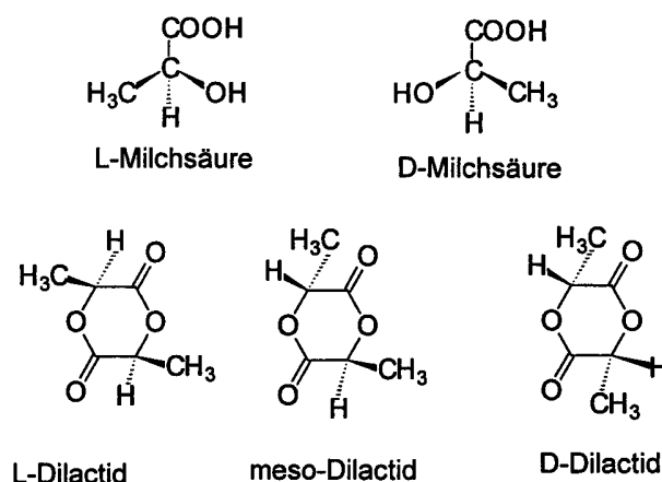
Schema 1: Chirale Milchsäuren und die daraus herstellbaren stereoisomeren zyklischen Diester
