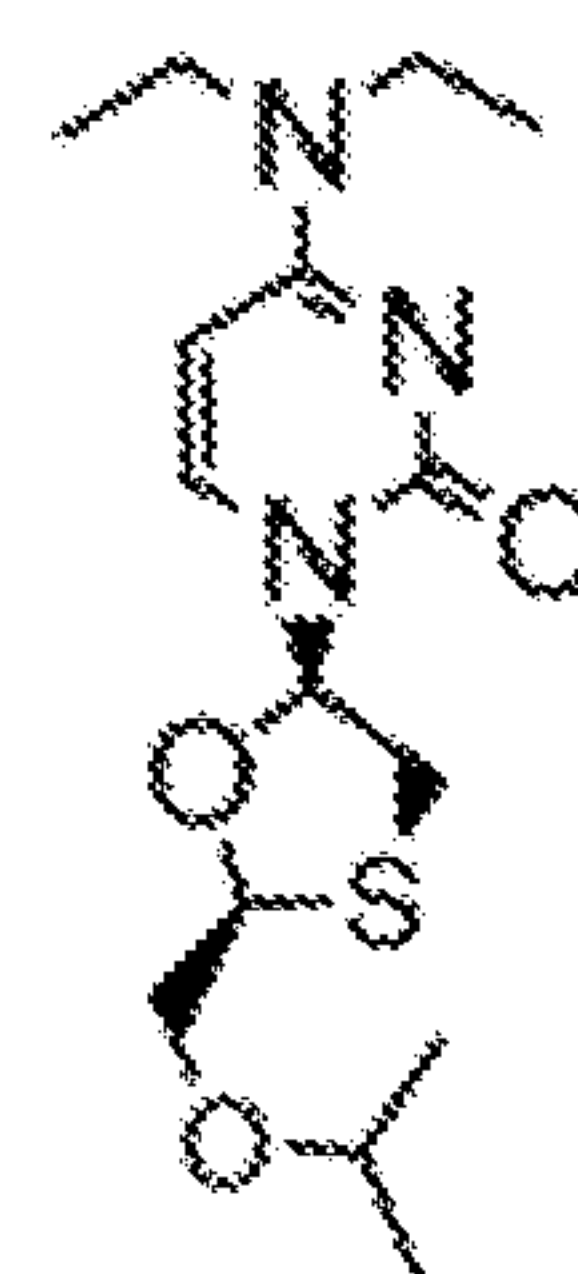
3tc-C7-3*,2,2
