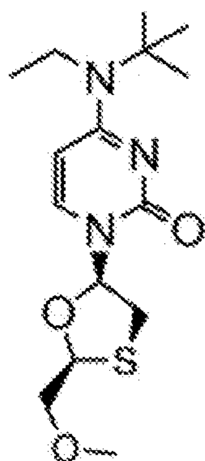
3tc-C7-1,2,4**
