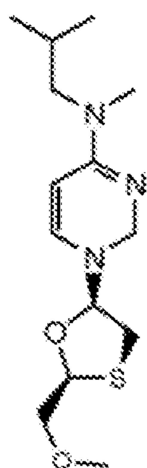
3tc-C6-1,4*,1
