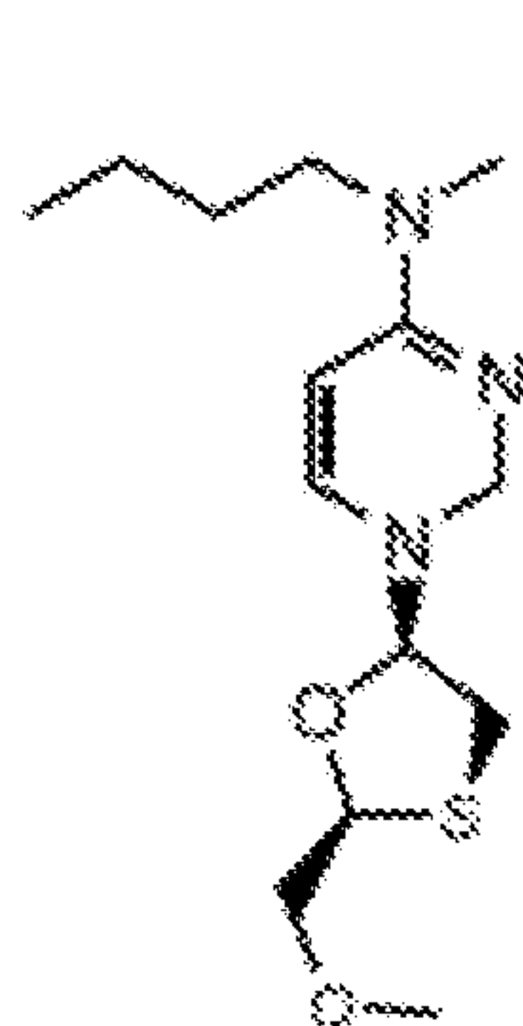
3tc-C6-1,4,1
