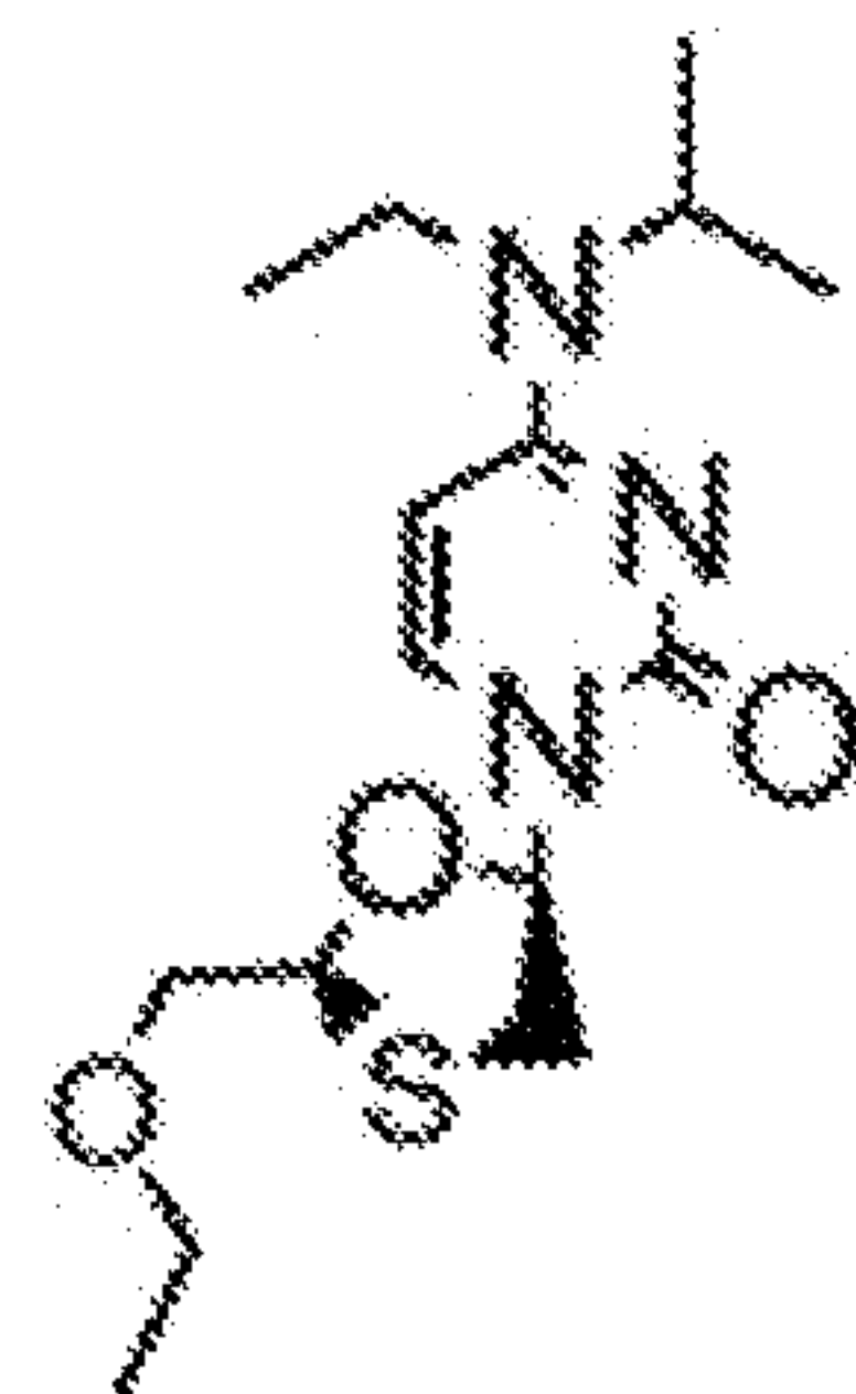
3tc-C7-2,2,3*
