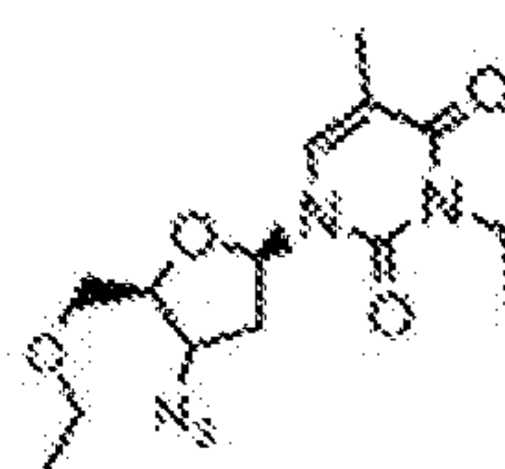
2-Et-AZT
