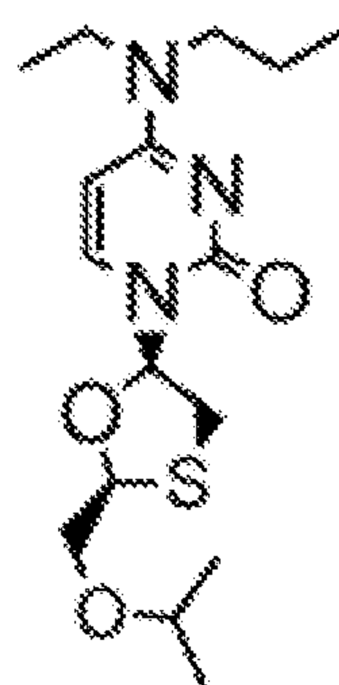
3tc-C8-3',2,3
