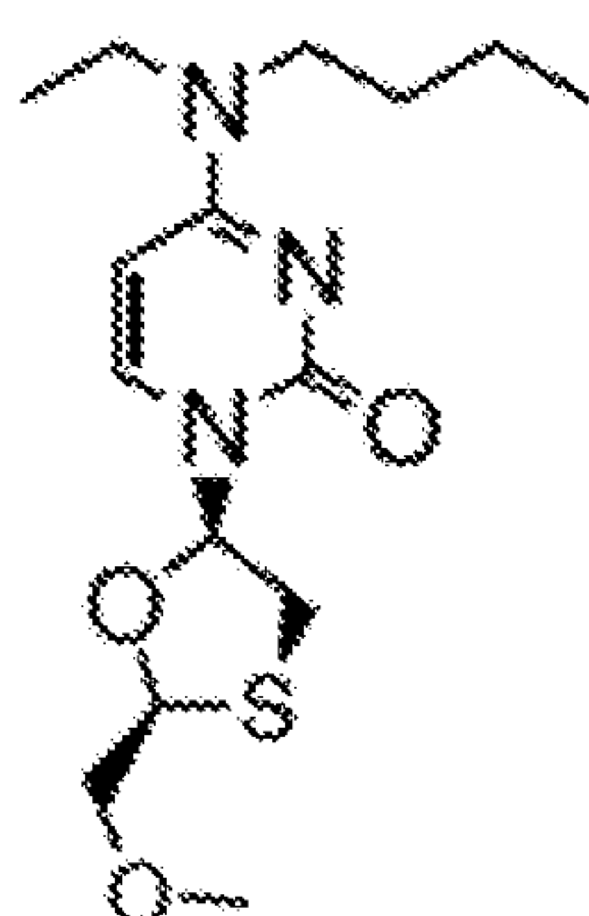
3tc-C7-1,2,4
