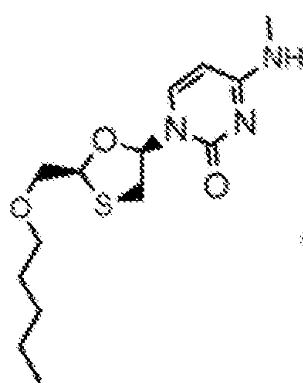
3tc-C6-5,1,0
