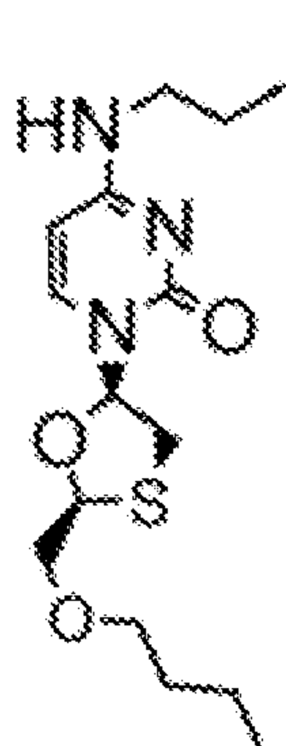
3tc-C7-4,0,3
