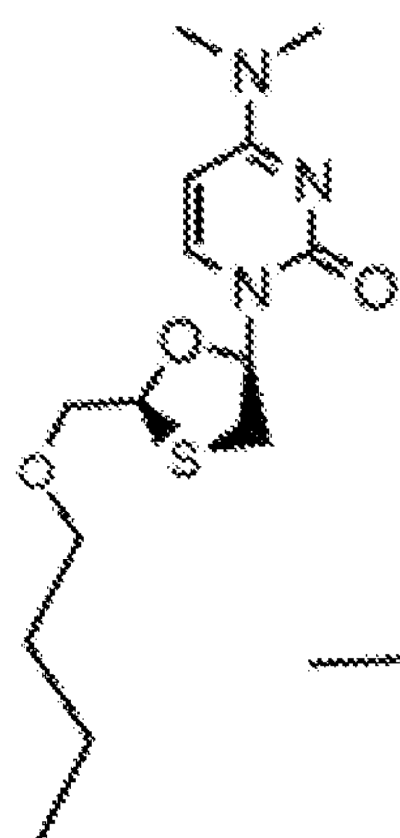
3tc-C6-4,1,1
