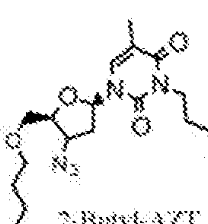
2-Butyl-AZT
