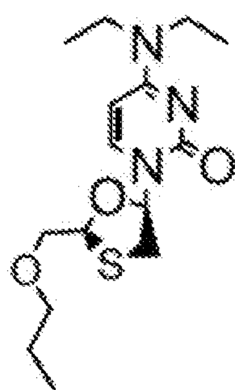
3tc-C7-3,2,2
