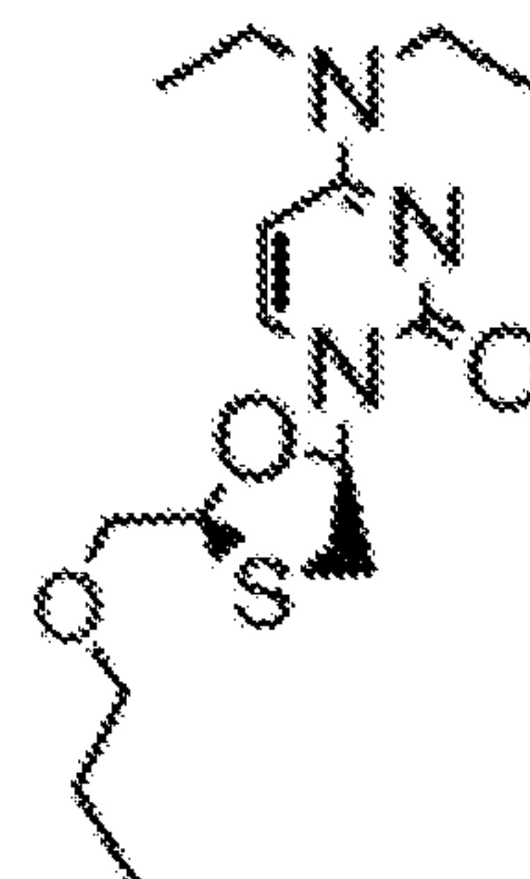
3tc-C7-3,2,2
