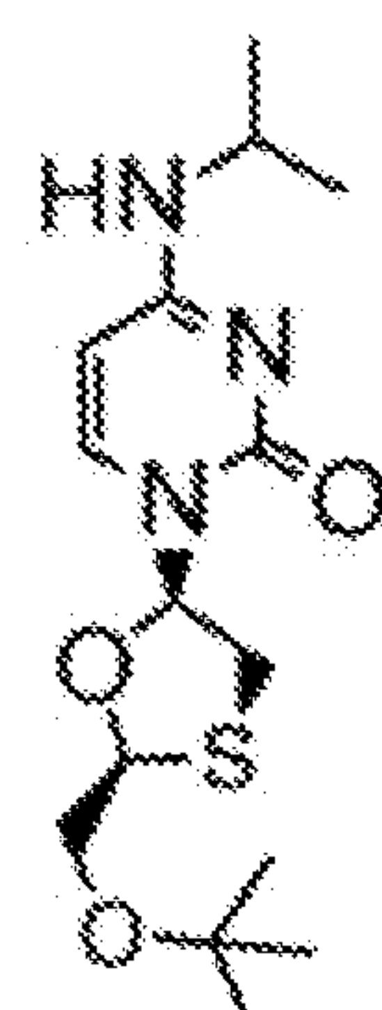
3tc-C7-4**,0,3
