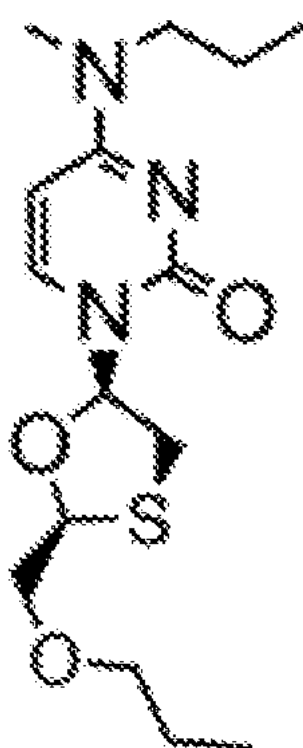
3tc-C7-3,1,3
