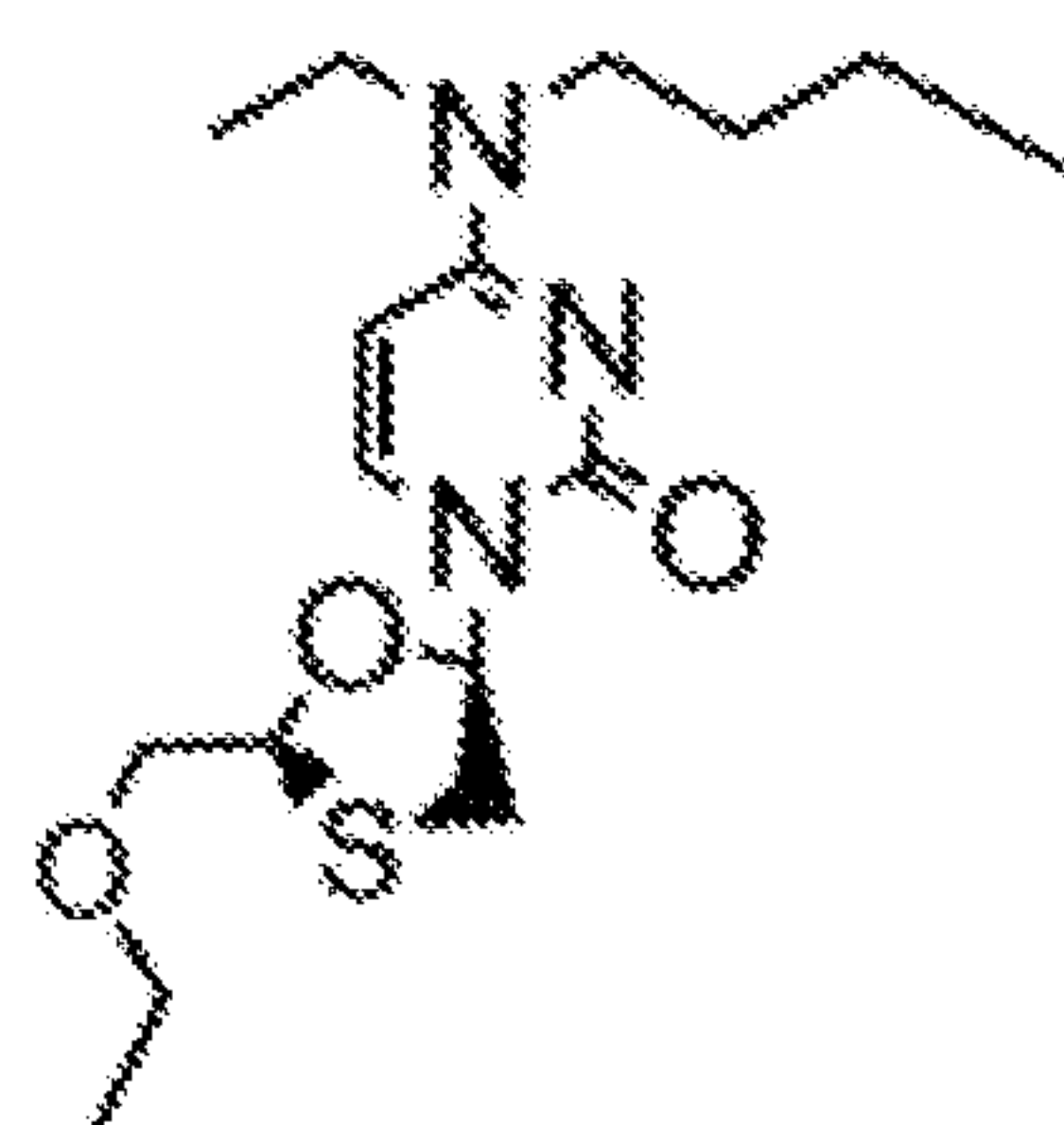
3tc-C8-2,2,4
