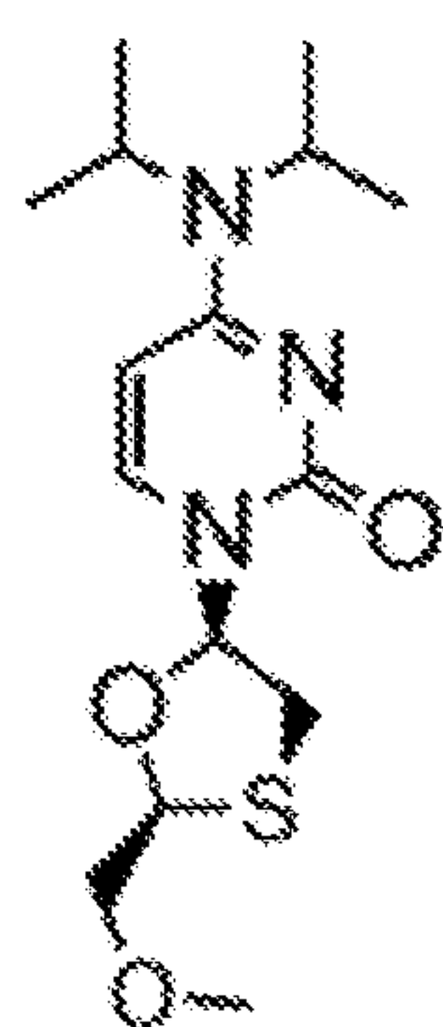
3tc-C7-1,3*,3*
