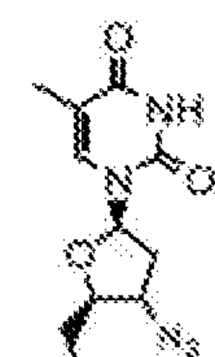
O-Me-AZT
