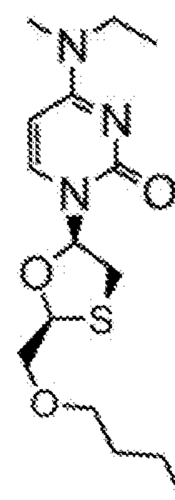
3tc-C7-4,1,2
