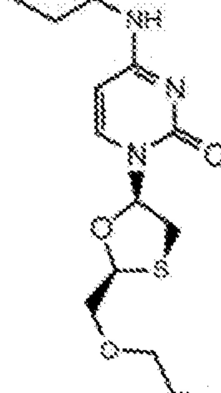
3tc-C6-3,3,0
