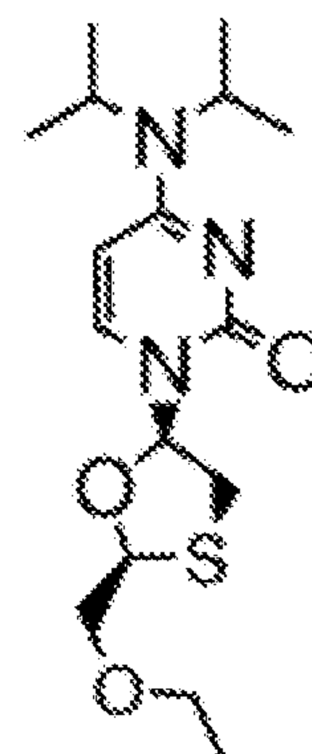
3tc-C8-2,3'3'
