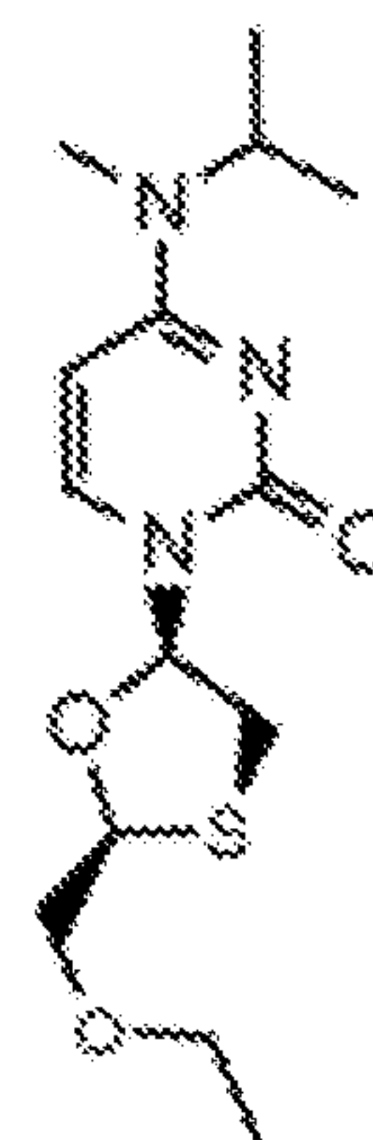
3tc-C6-2,1,3*
