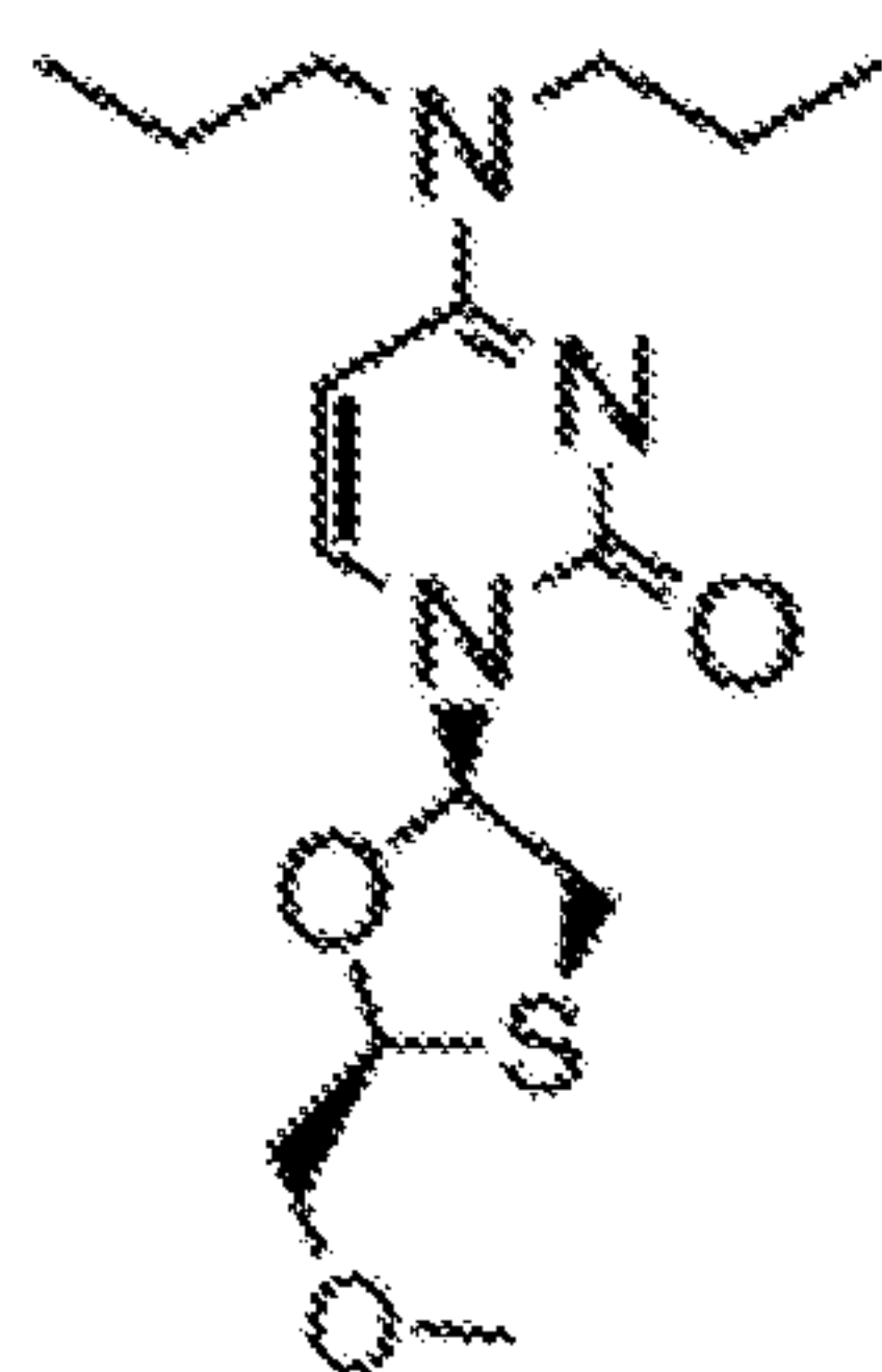
3tc-C7-1,3,3
