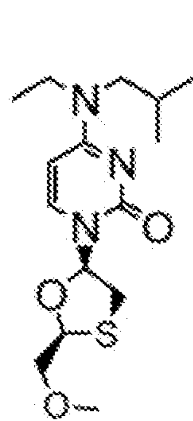
3tc-C7-1,2,4*
