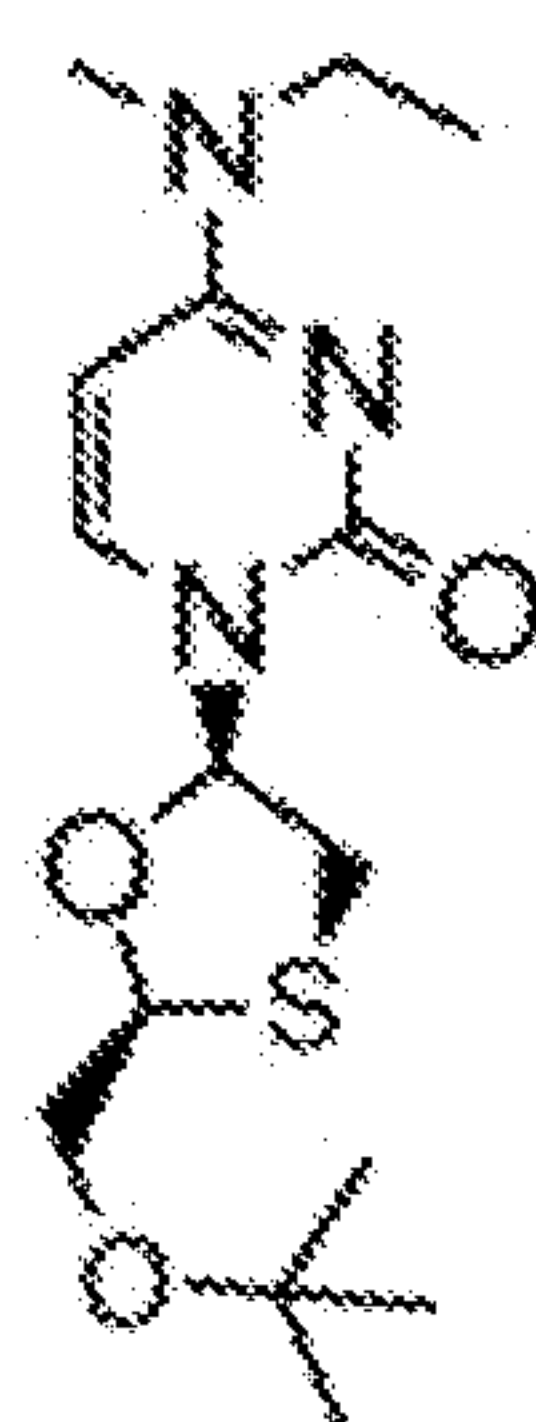
3tc-C7-4**,1,2
