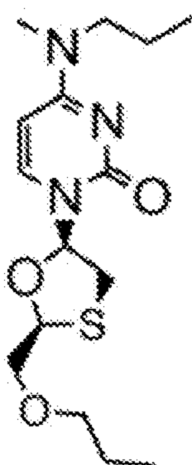
3tc-C7-3,1,3
