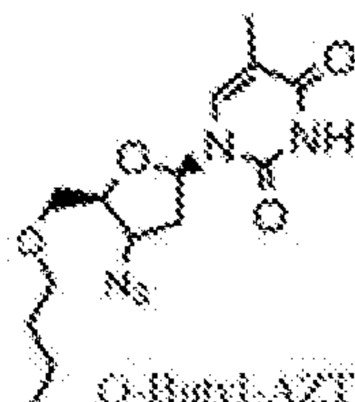
O-Butyl-AZT
