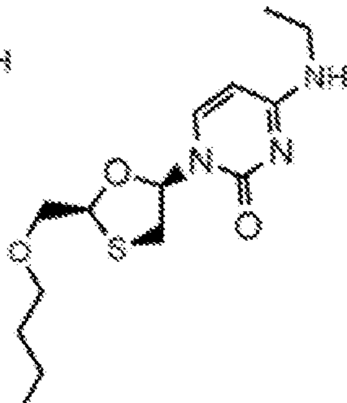
3tc-C6-4,2,0
