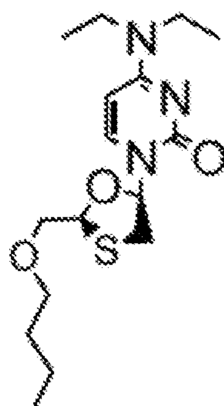
3tc-C8-4,2,2
