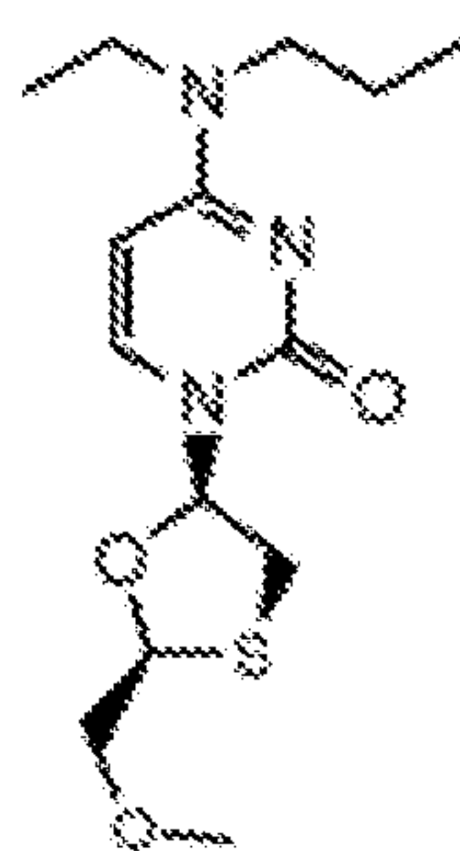
3tc-C6-1,2,3
