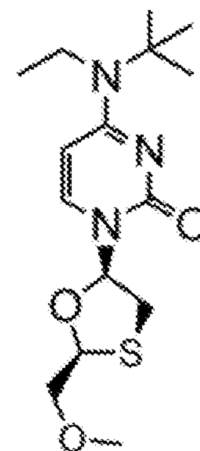
3tc-C7-1,2,4**
