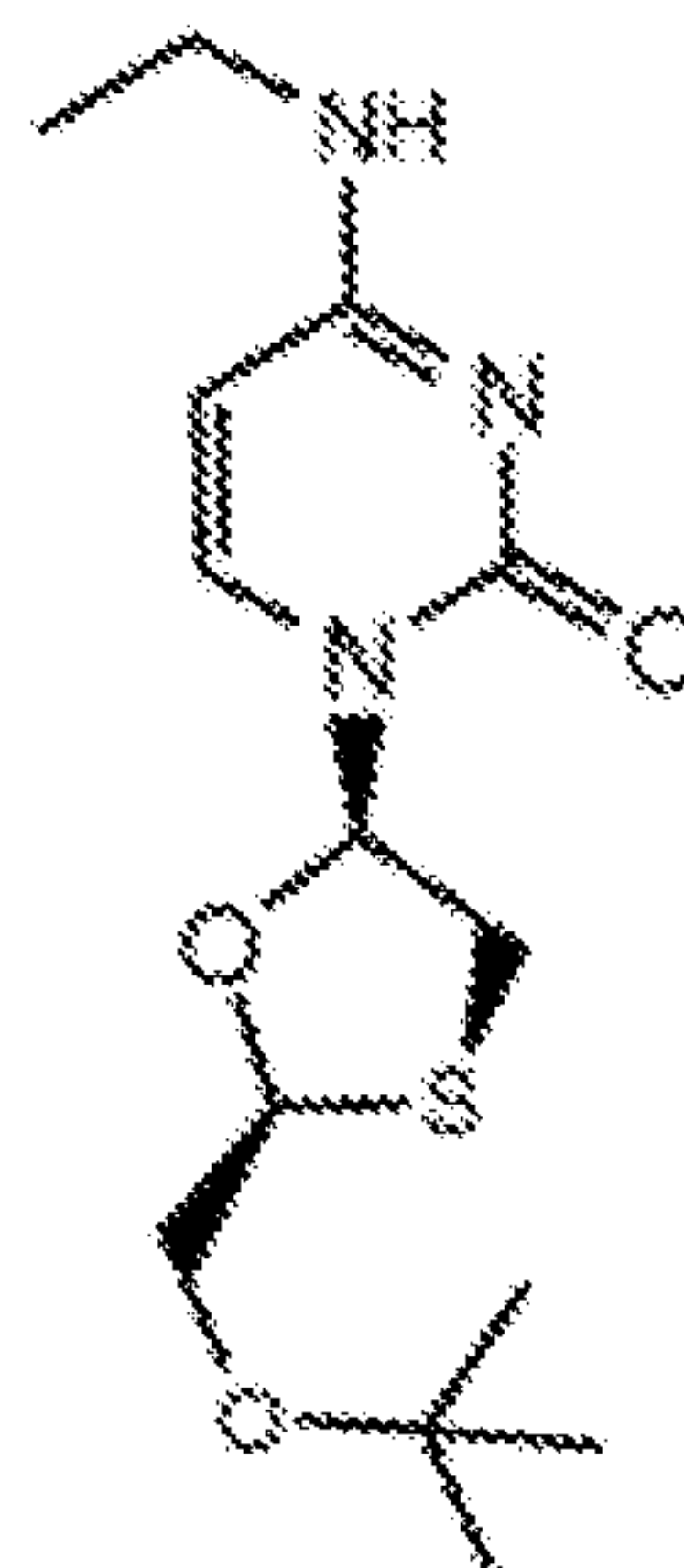
3tc-C6-4**,2,0
