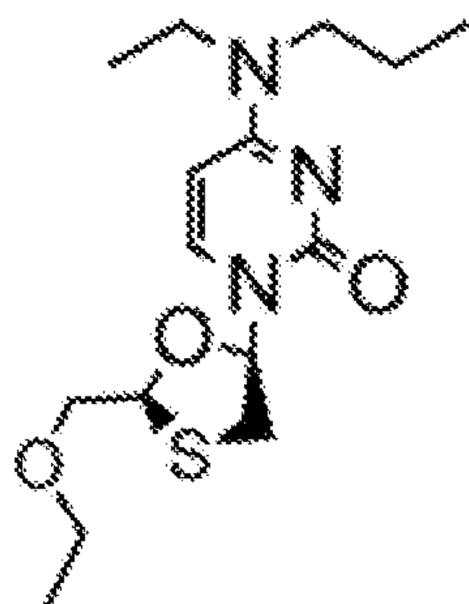
3tc-C7-2,2,3
