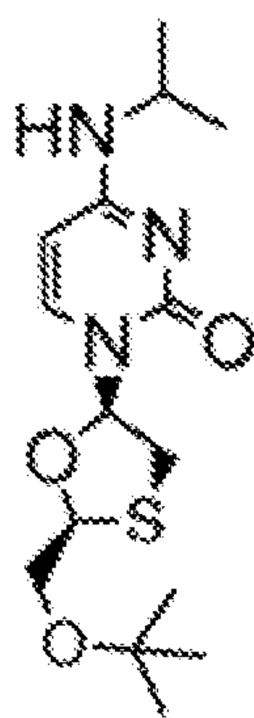
3tc-C7-4**,0,3
