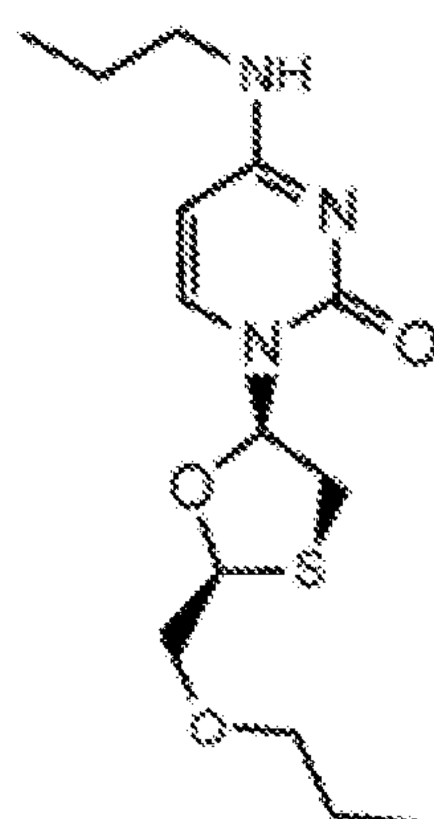
3tc-C6-3,3,0
