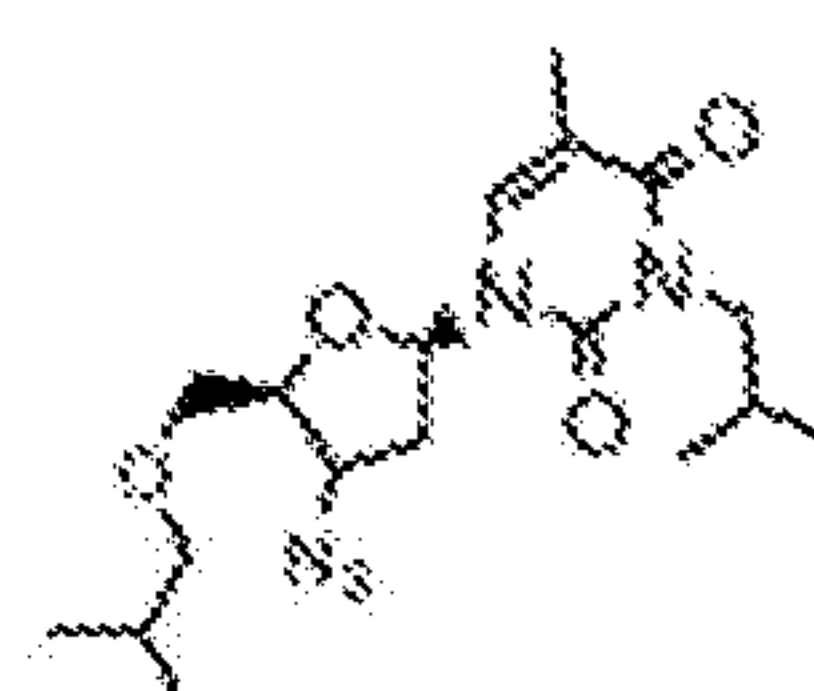
2-isobutyl-AZT
