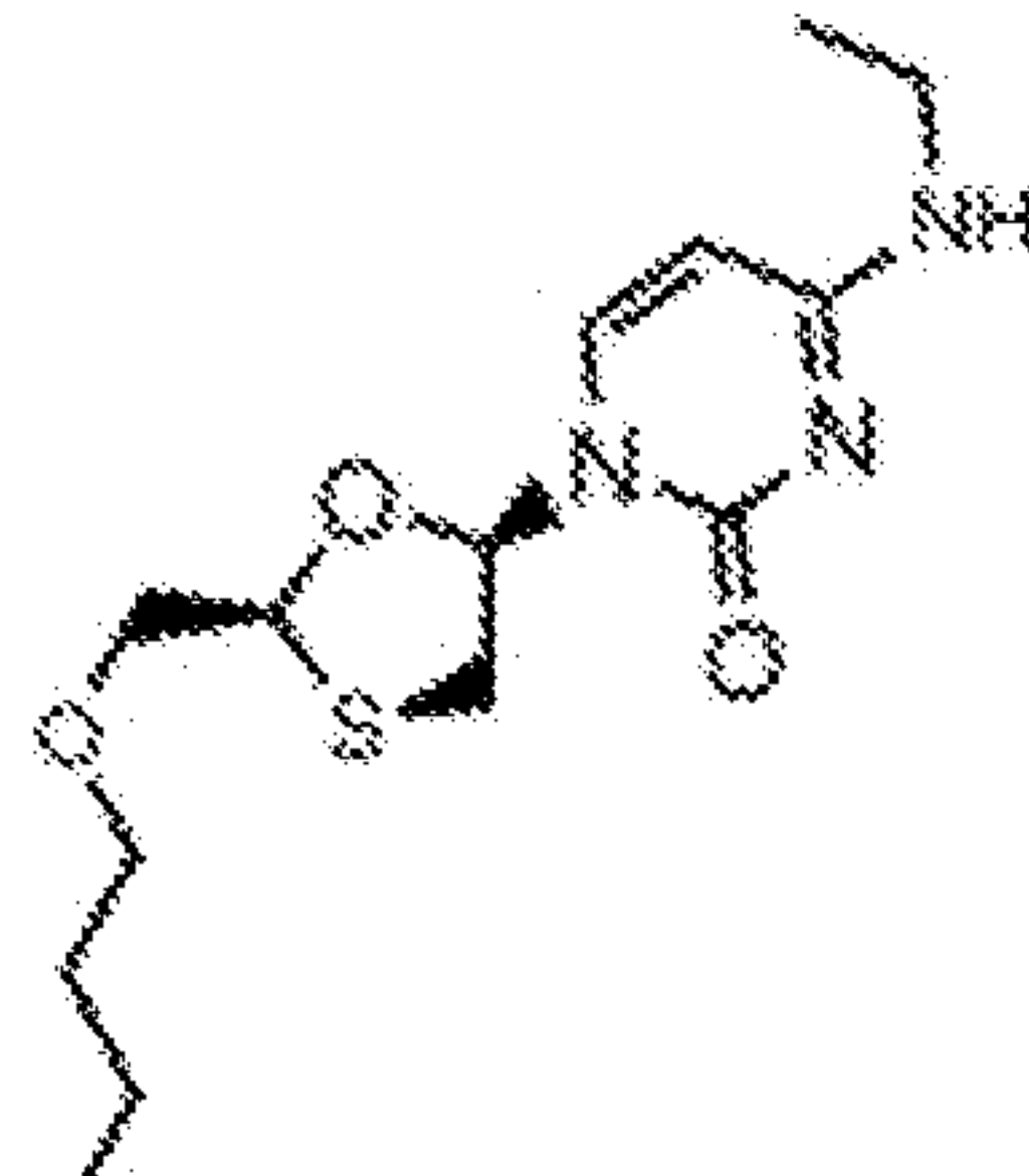
3tc-C6-4,2,0
