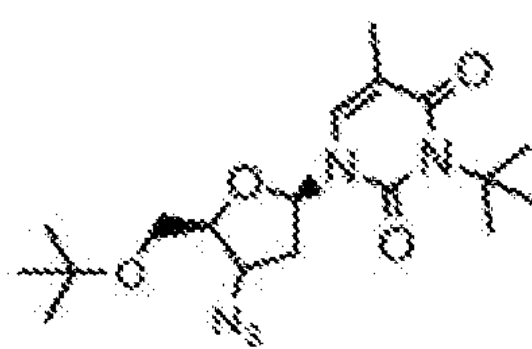
2-tert-butyl-AZT
