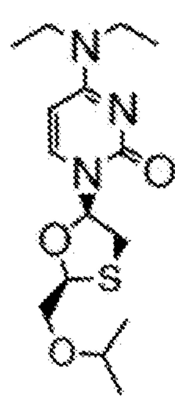
3tc-C7-3*,2,2
