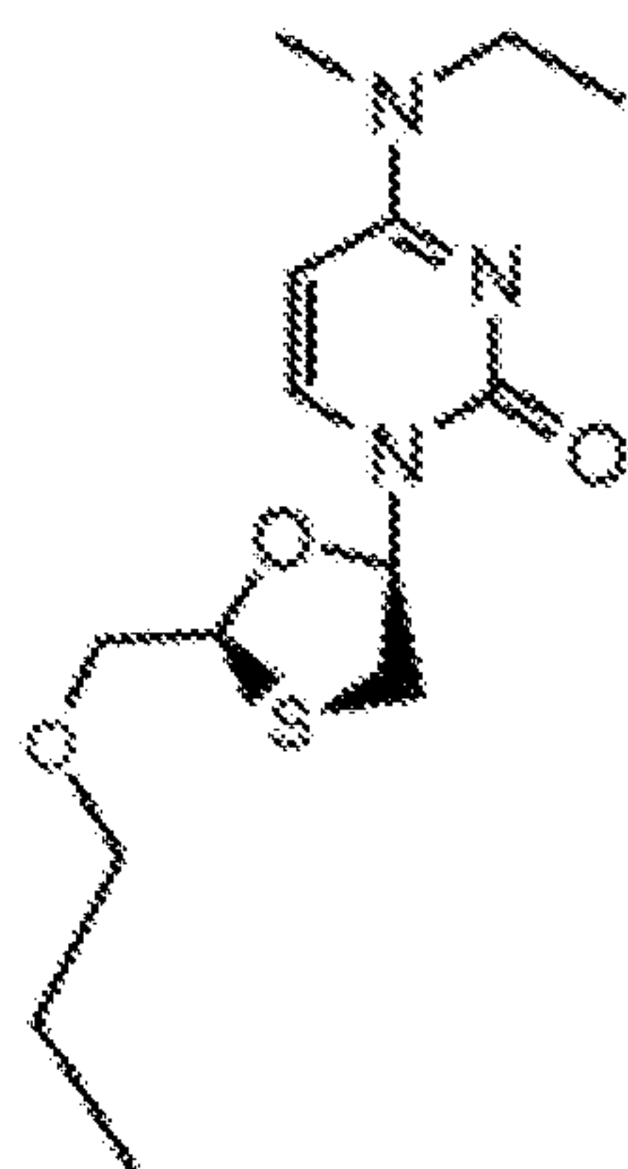
3tc-C6-3,1,2
