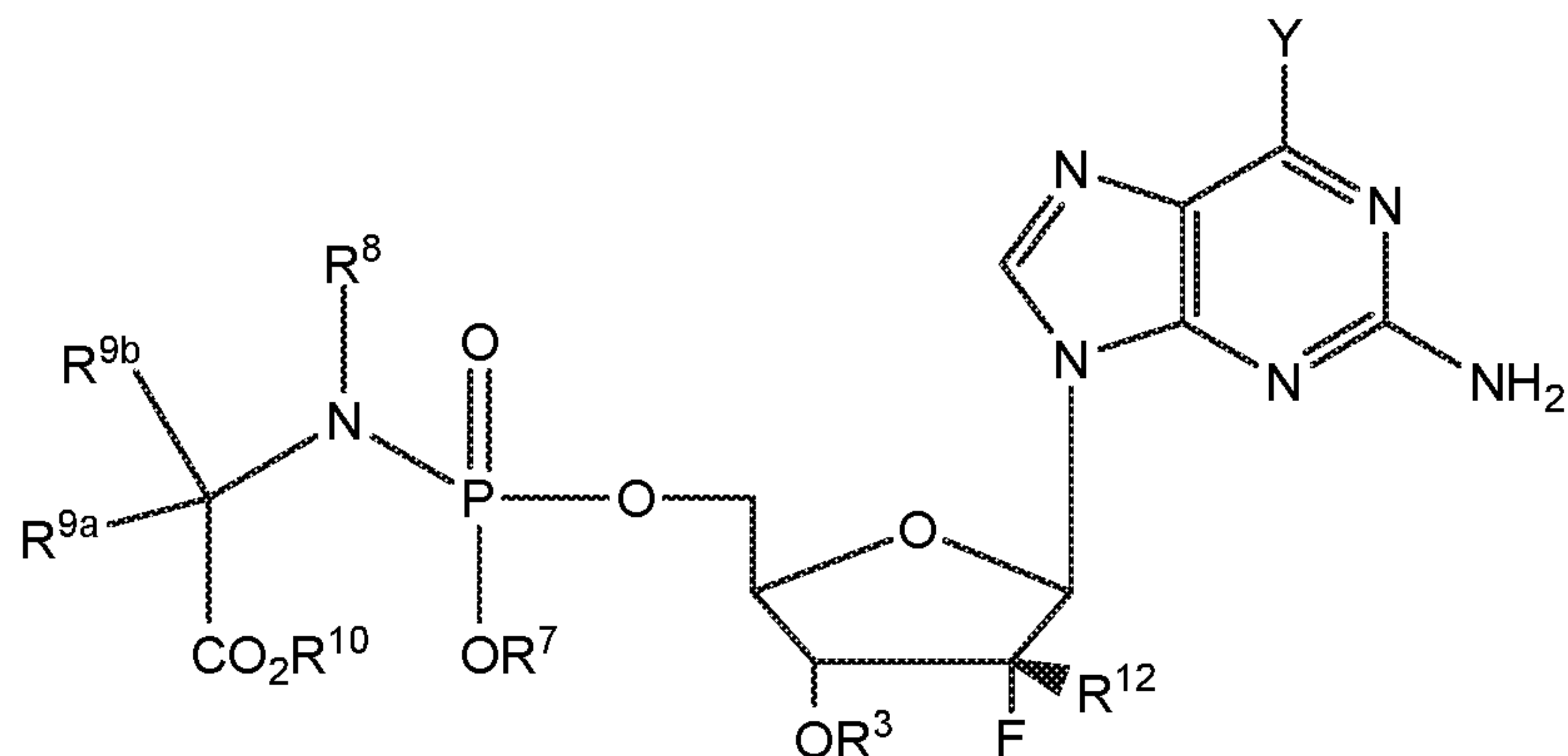
Formula Ic
