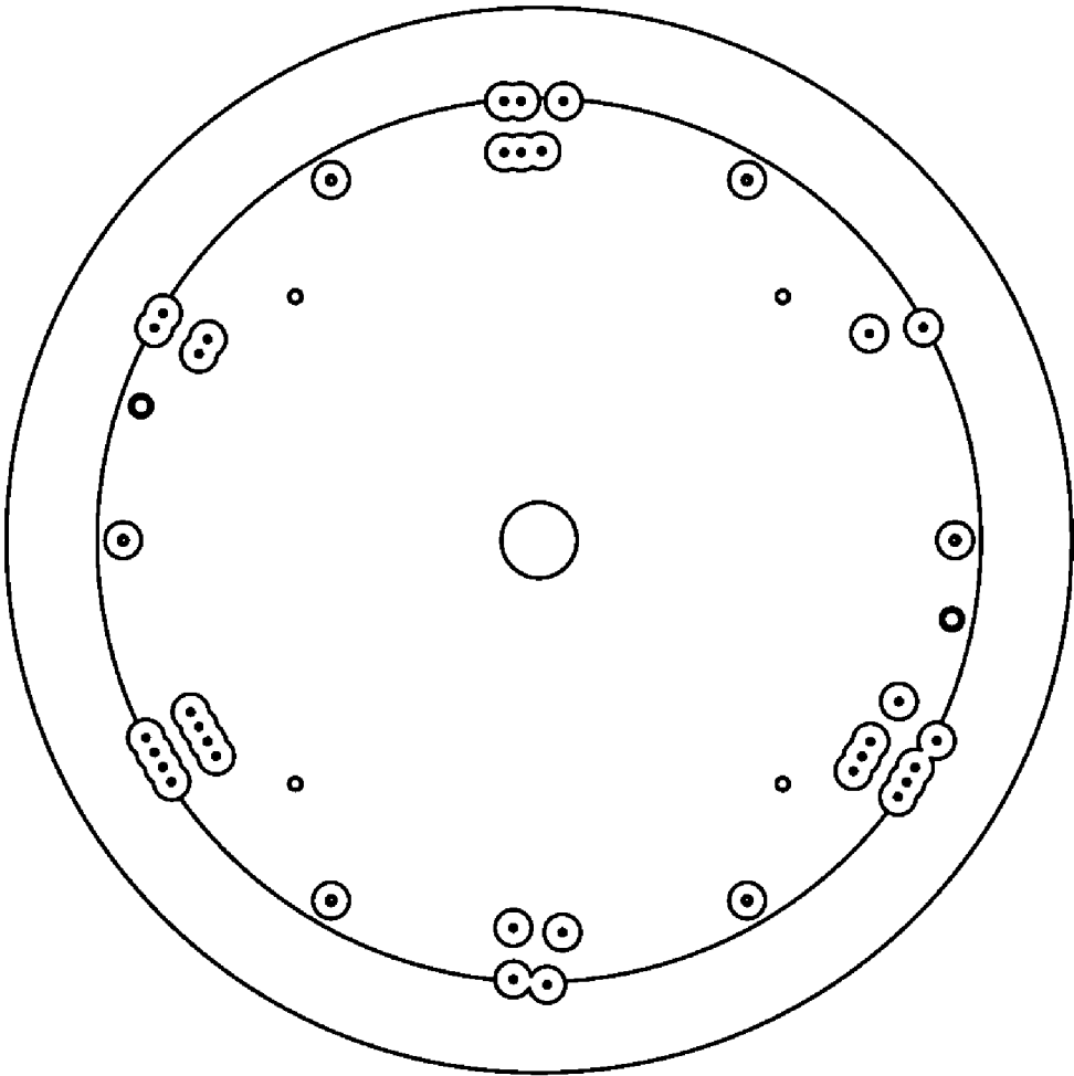
【後視圖】
