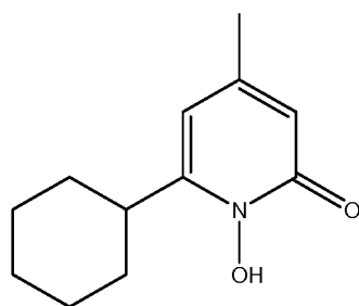
Ciclopirox
