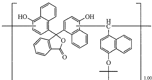
Novolak Resin 17
