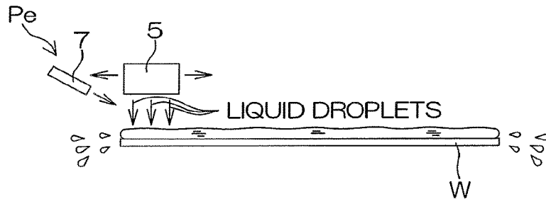
FIG. 7D RINSING STEP
