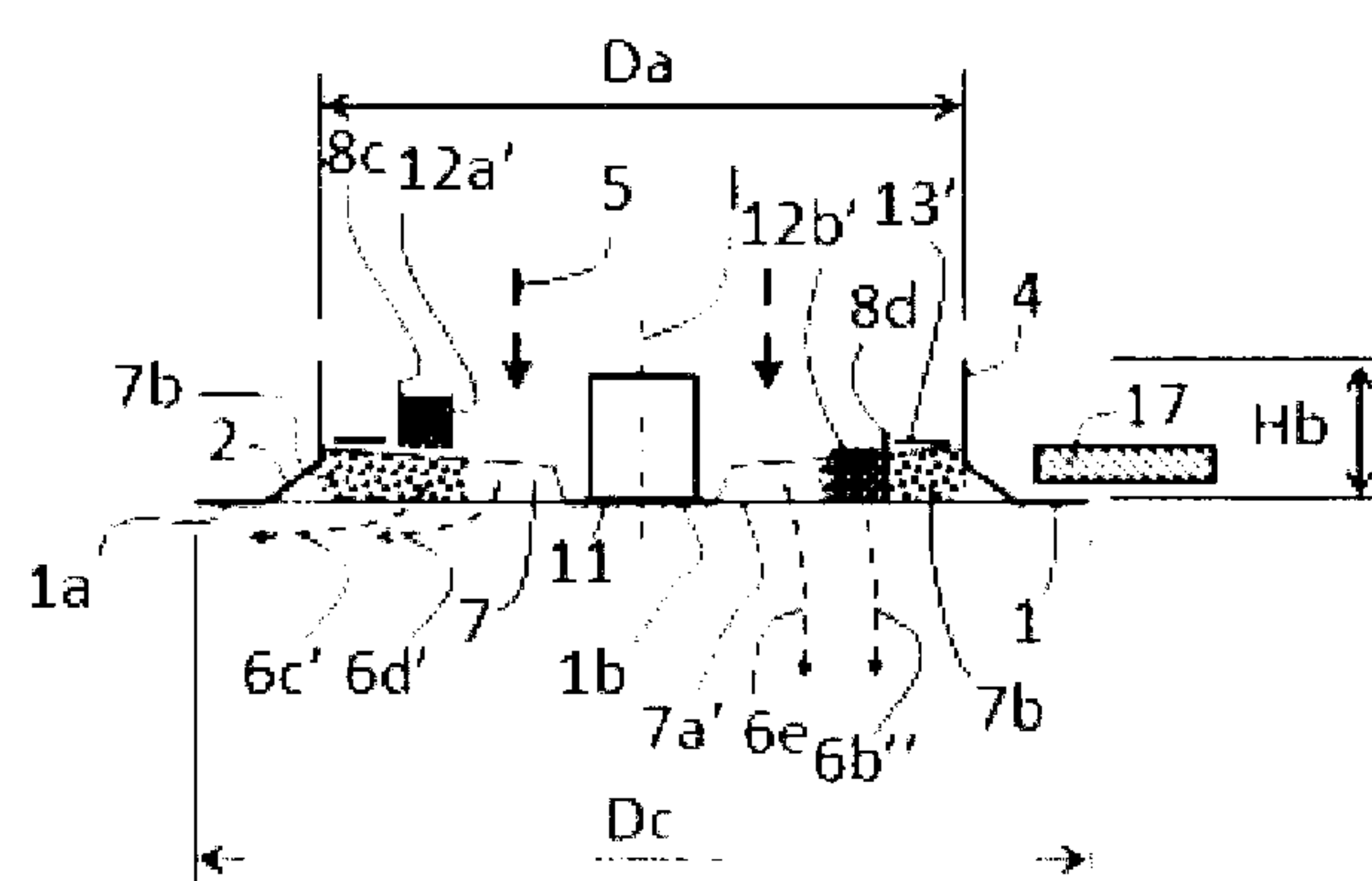
b) Section A-A
