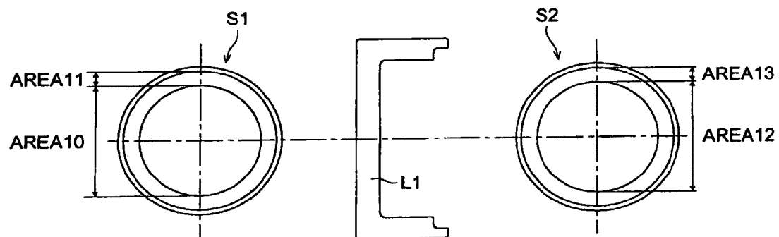
FIG. 6 (a) FIG. 6 (b) FIG. 6 (c)
