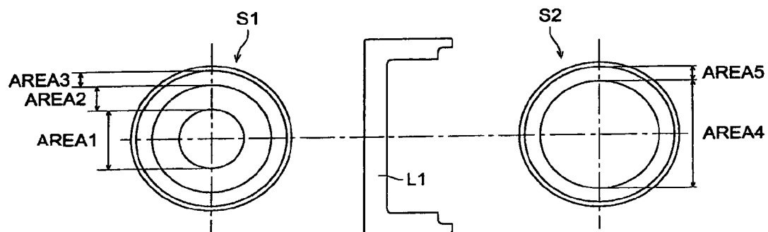
FIG. 2 (a) FIG. 2 (b) FIG. 2 (c)
