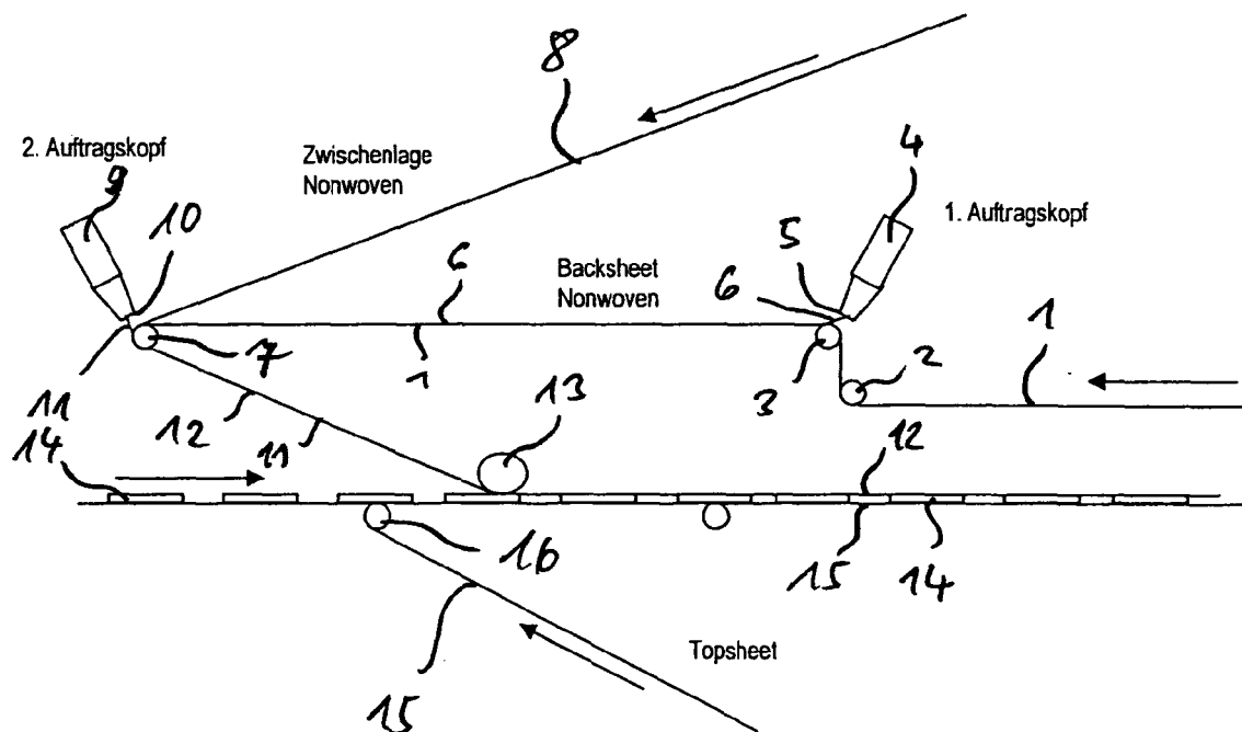
Skizze der Bahnführung beim doppelten Auftrag – (alternativer Wäscheschutz)
