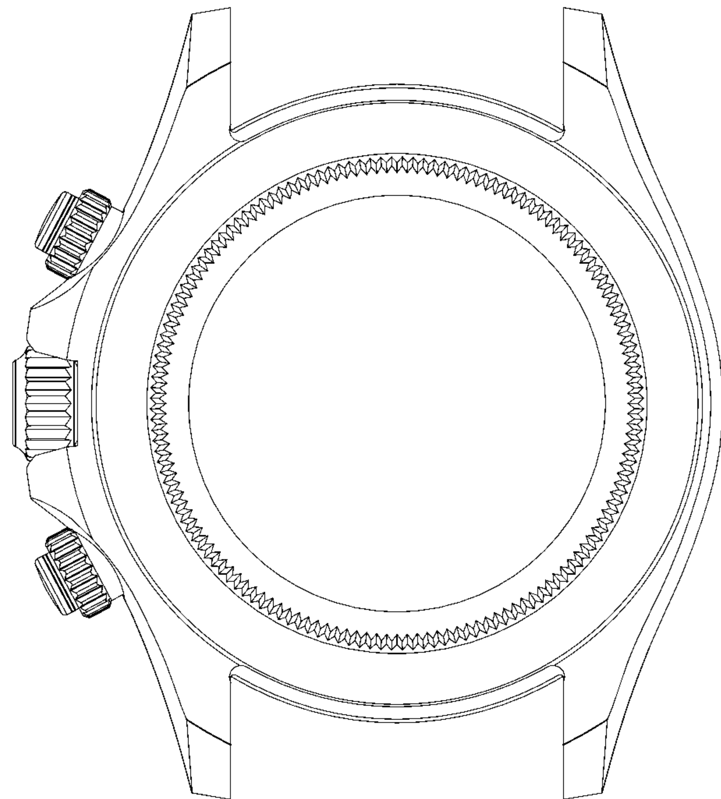
【後視圖】
