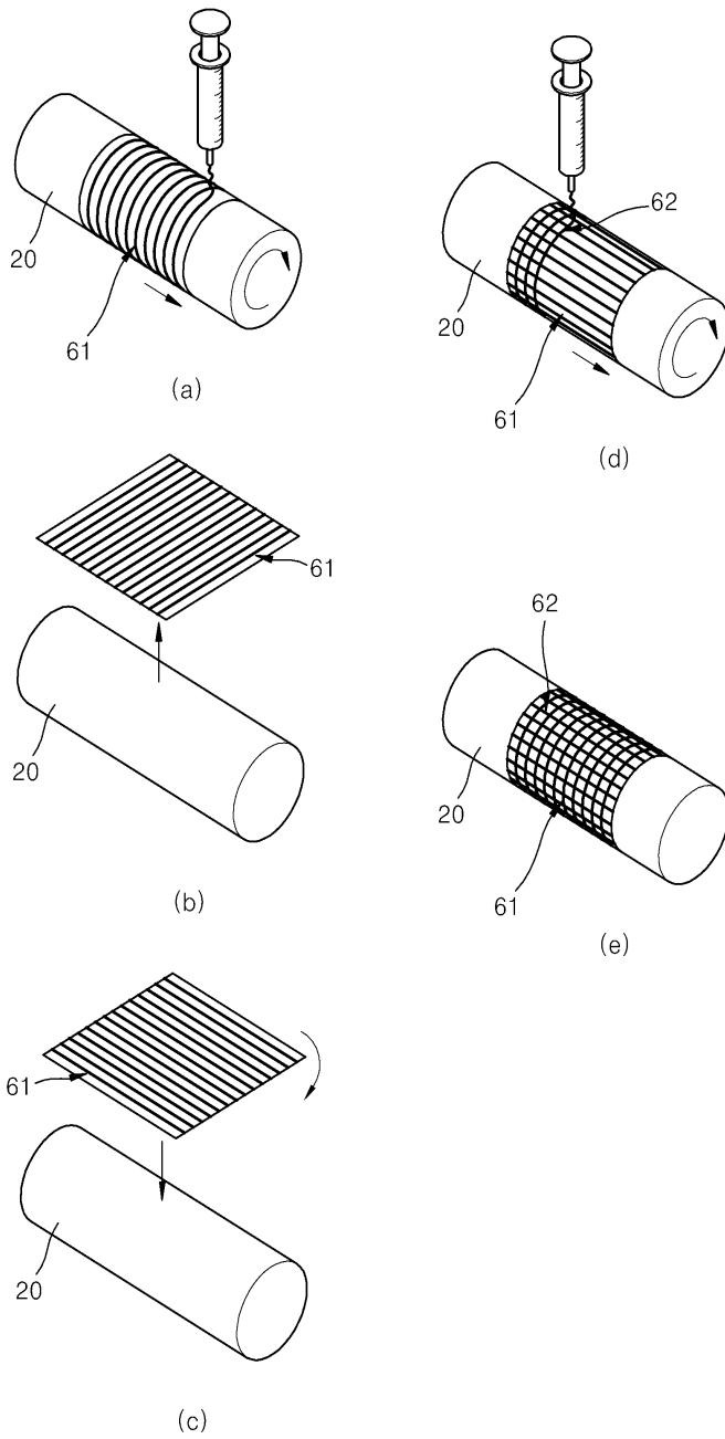
도면5
