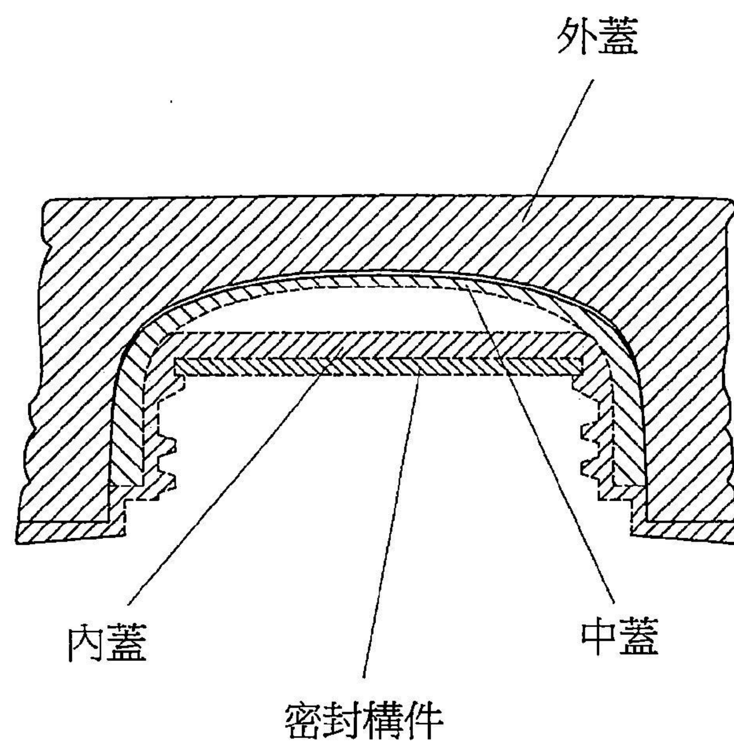
顯示各部之名稱的參考 A - A 線剖面圖
