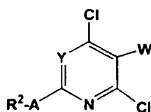
(VI-a)
