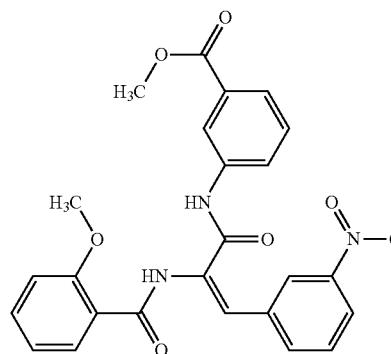
methyl 3[(2-(2-methoxybenzoyl)amino)-3-(3-nitrophenyl)acryloyl]amino]benzoate
