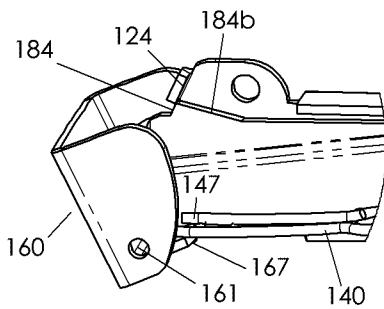
FIG. 25A
