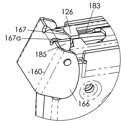
FIG. 32A
