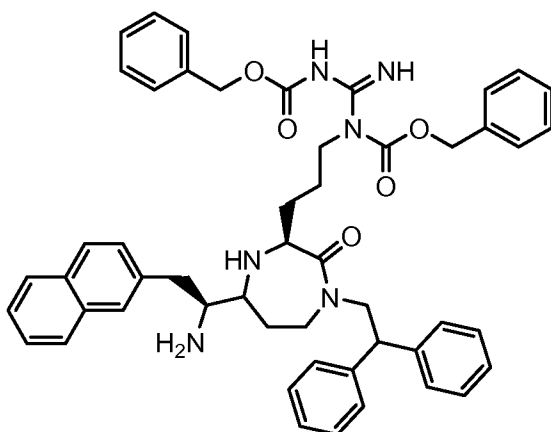
78 bis (Cbz) 1-(3-((2 S ,7 RS )-7-(( S )-1-amino-2-(naphthalen-2-yl)ethyl)-4-(2,2-diphenylethyl)-3-oxo-1,4-diazepan-2-yl)propyl)guanidine
