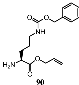
90 ( S )-allyl 2-amino-5-(benzyloxycarbonylamino)pentanoate
