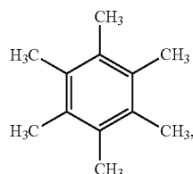
hexamethylbenzene
