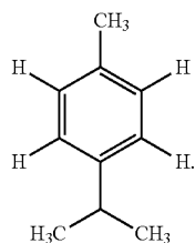
p-cymene
