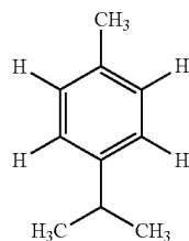
p-cymene
