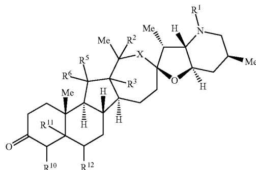
(I-AA)
