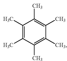
hexamethylbenzene
