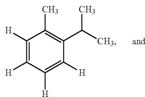
m-cymene
