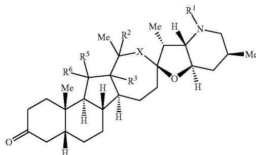
(I-BB)
