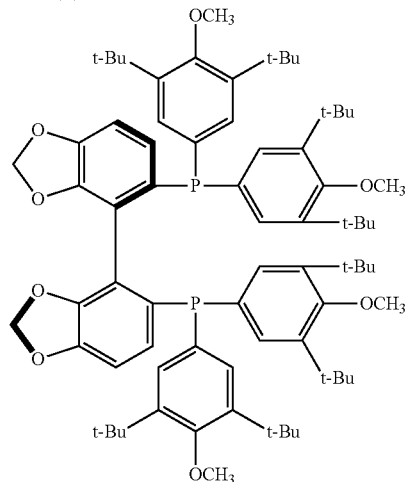
L(R)-DTBM-SEGPHOS
