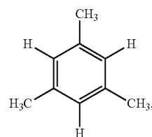
mesitylene
