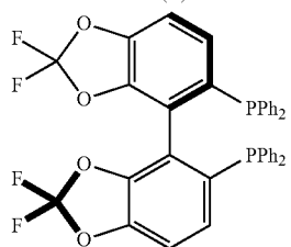
(R)-DIFLUORPHOS
