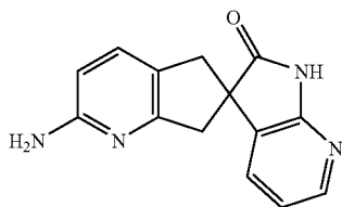
( \pm )-2-Amino-5,7-dihydrospiro[cyclopenta[b]pyridine-6,3'-pyrrolo[2,3-b]pyridin]-2'-(1'H)-one
