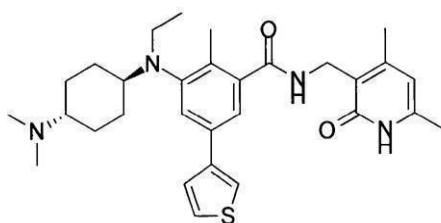
化合物156
