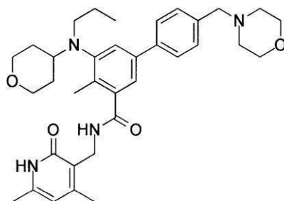
化合物59
