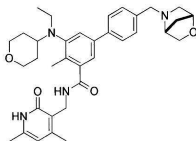
化合物67
