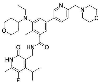
化合物197
