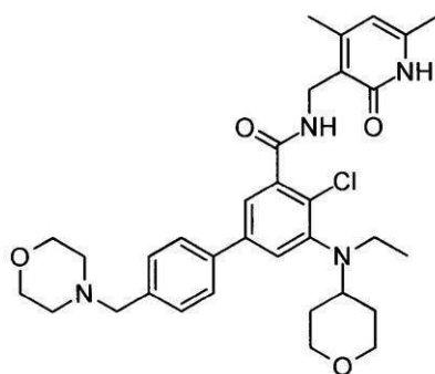
化合物178
