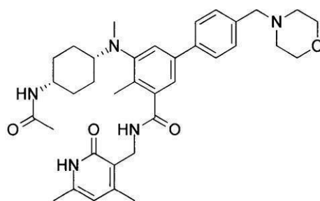
化合物20
