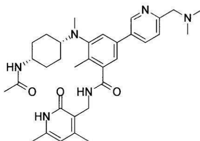
化合物55
