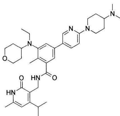
化合物193
