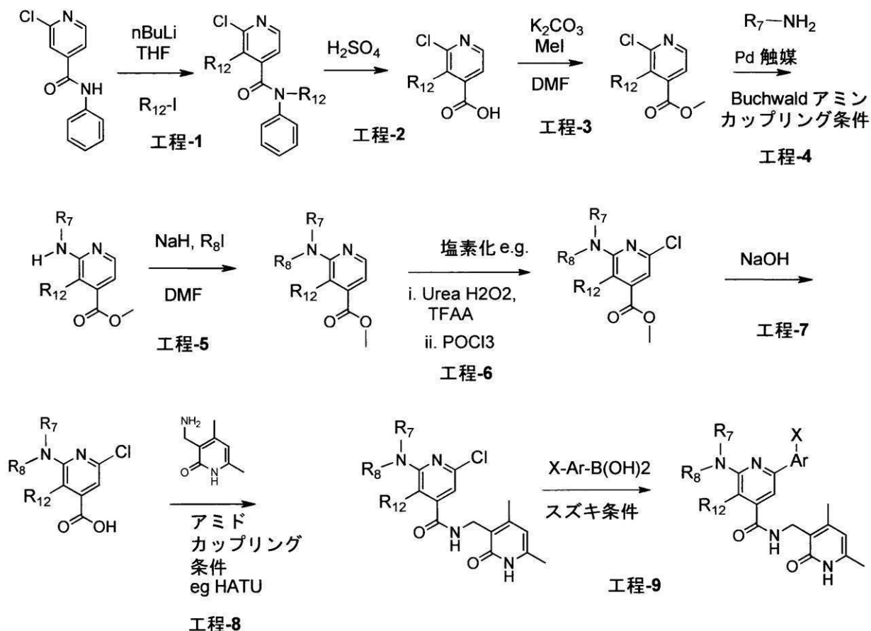
スキーム8
