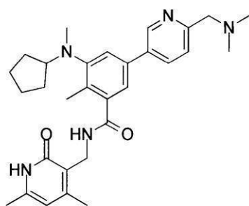
化合物35
