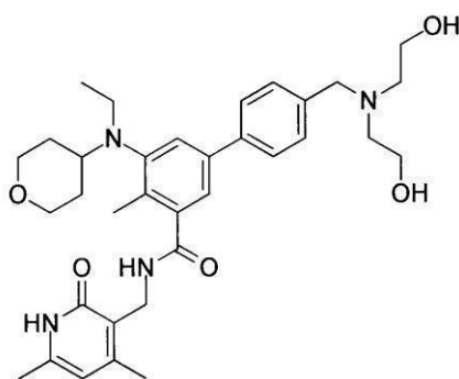
化合物100
