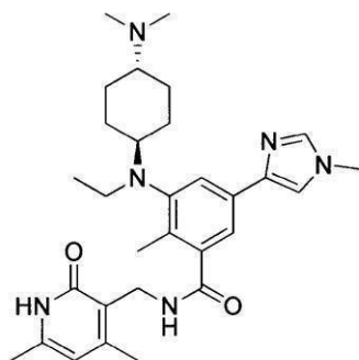
化合物180
