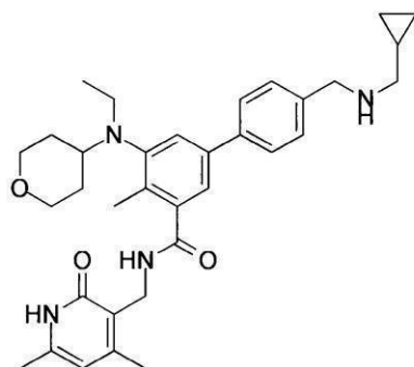
化合物93
