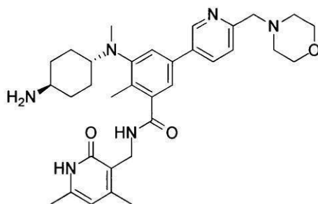
化合物50
