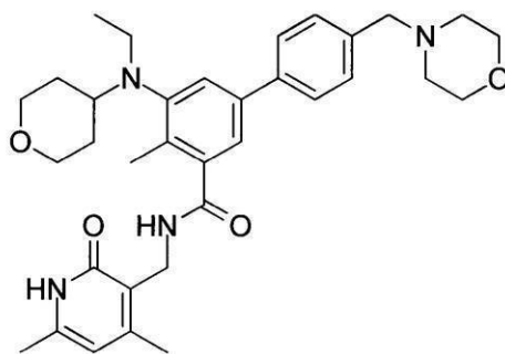
化合物44
