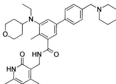
化合物75
