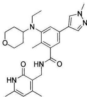
化合物109
