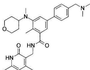
化合物13
