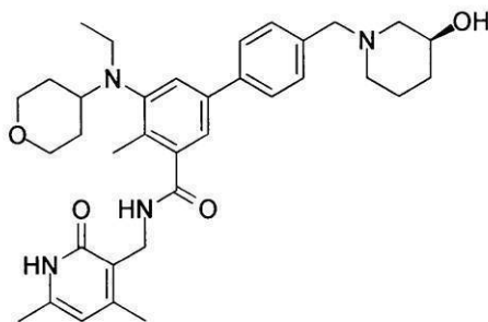
化合物76
