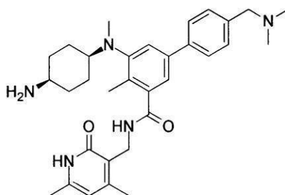
化合物47
