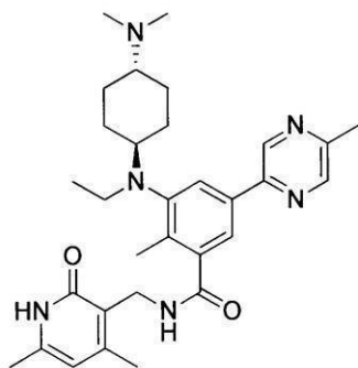
化合物175
