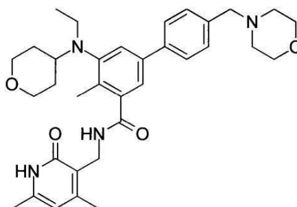
化合物44
