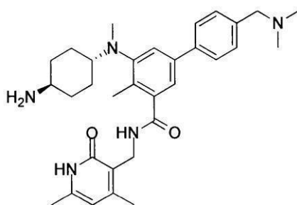
化合物108
