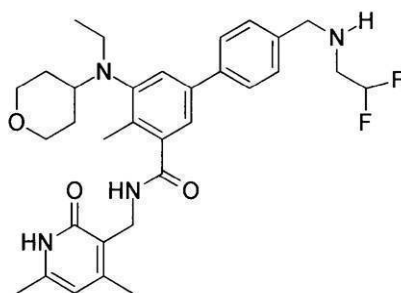
化合物103
