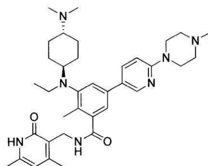
化合物170
