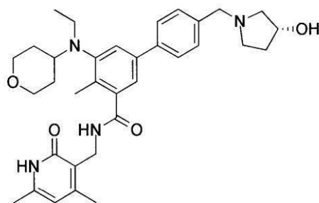
化合物71
