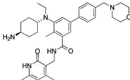
化合物128
