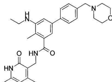
化合物117
