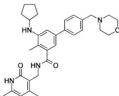
化合物 4
