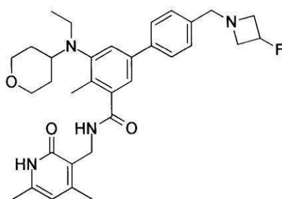
化合物84
