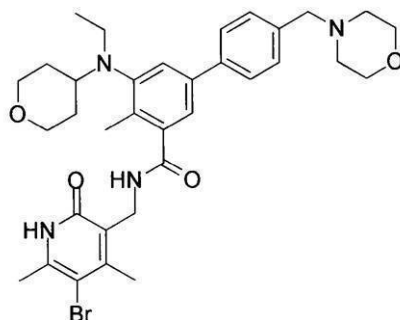
化合物177
