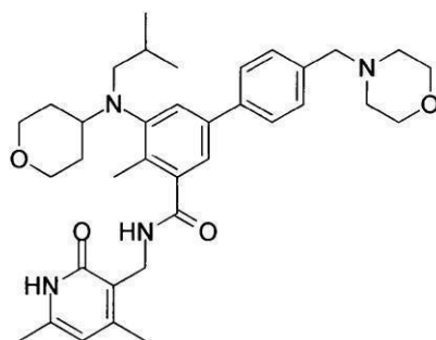
化合物60
