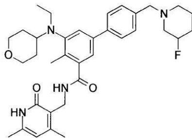
化合物79
