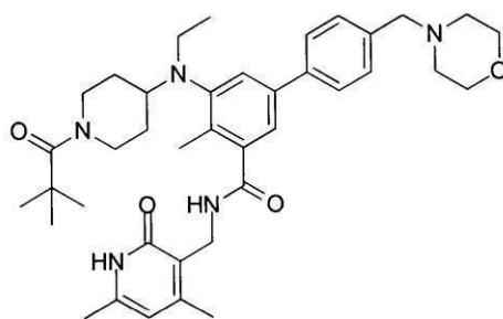
化合物127
