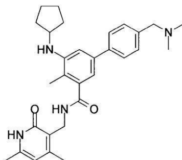
化合物3
