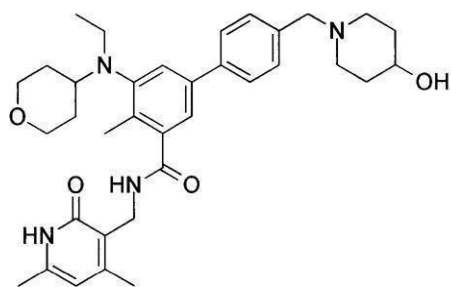
化合物78
