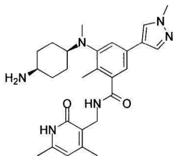
化合物46
