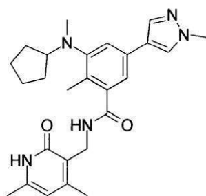
化合物19
