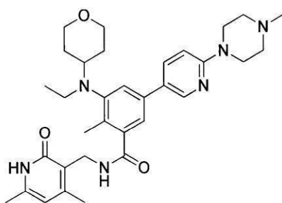
化合物171
