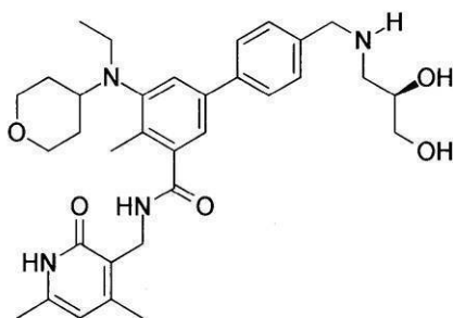
化合物95
