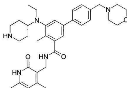
化合物126
