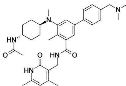
化合物39
