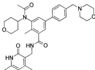
化合物119
