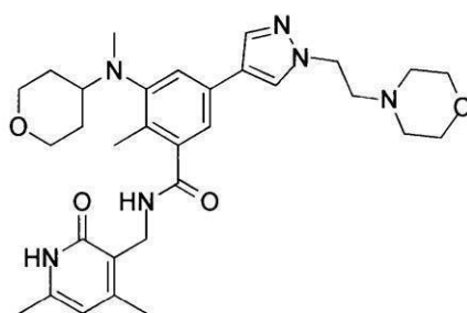
化合物 8
