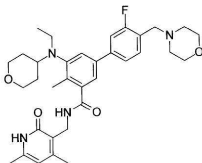
化合物120
