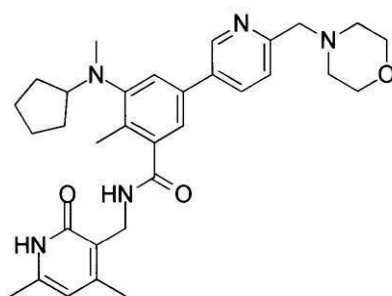
化合物17
