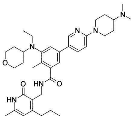
化合物194
