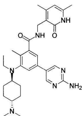
化合物154
