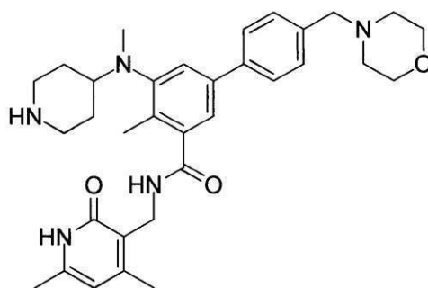
化合物11
