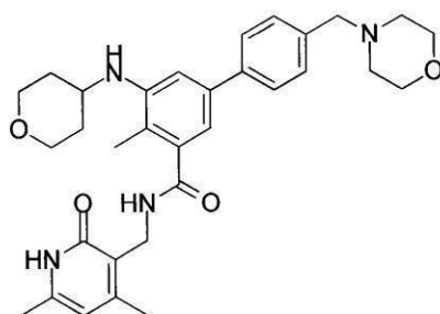
化合物116
