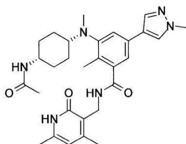
化合物22
