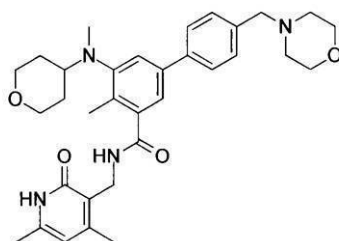
化合物12
