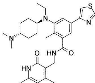
化合物166
