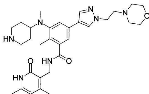
化合物25
