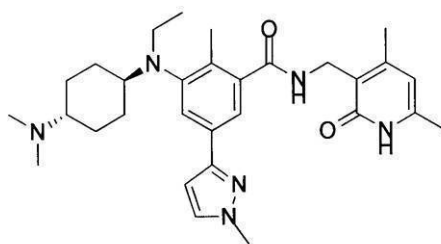
化合物161
