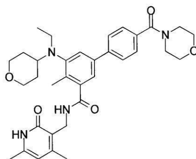
化合物123
