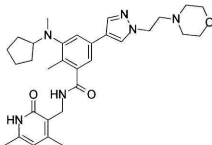
化合物18
