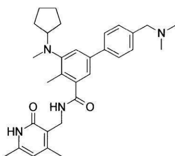
化合物 1
