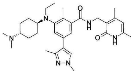
化合物165
