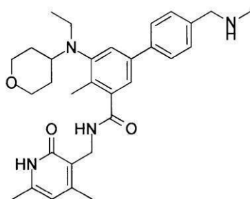
化合物90
