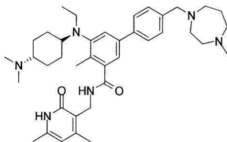
化合物146
