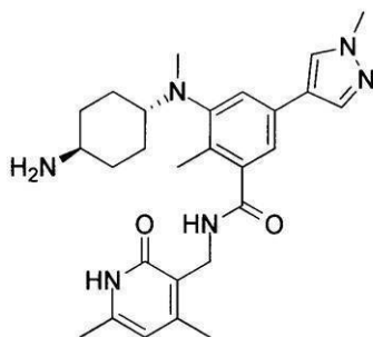
化合物45
