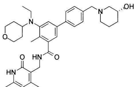
化合物77
