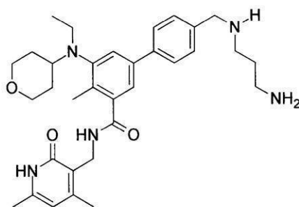
化合物102
