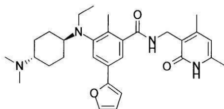
化合物152
