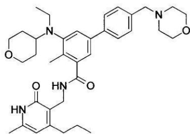
化合物176
