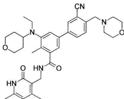
化合物140
