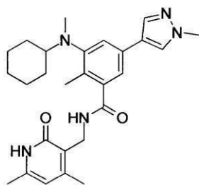
化合物10
