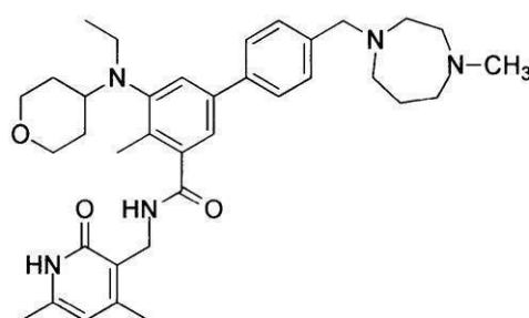
化合物87
