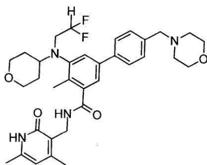
化合物144
