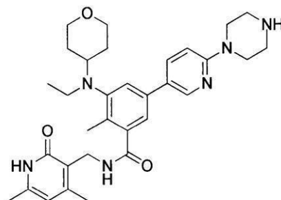
化合物173
