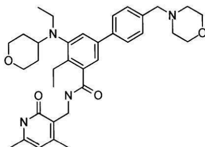
化合物139
