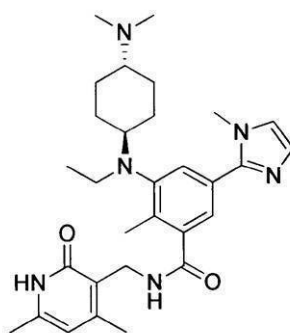
化合物169
