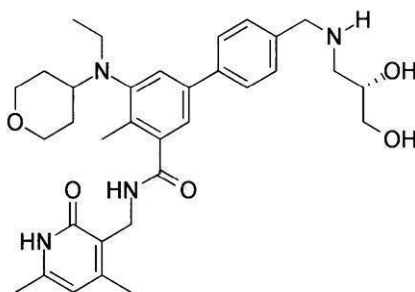
化合物96
