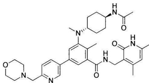
化合物54
