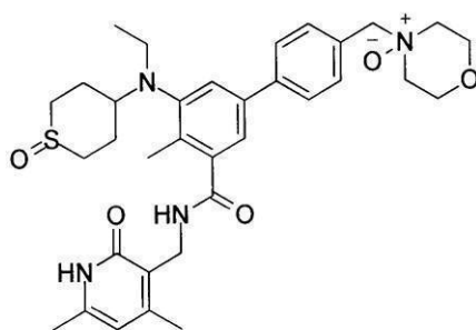
化合物135
