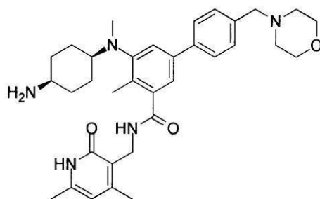
化合物42
