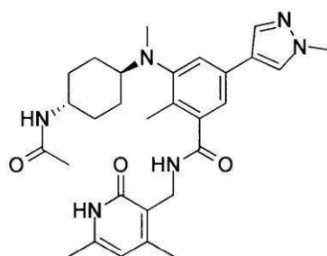
化合物23
