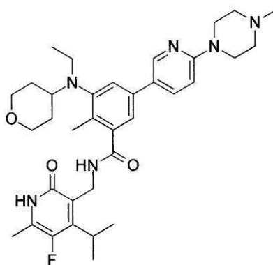
化合物196
