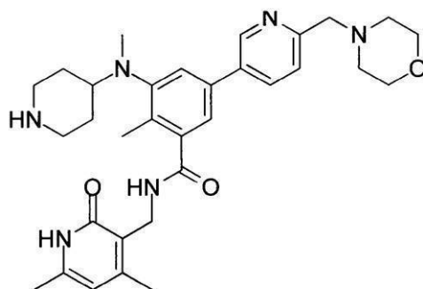
化合物24
