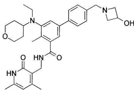
化合物83
