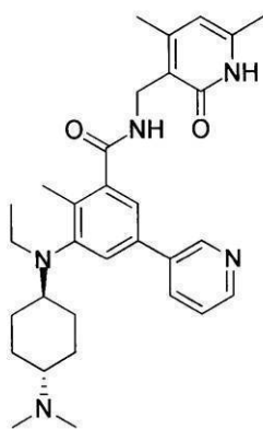
化合物162
