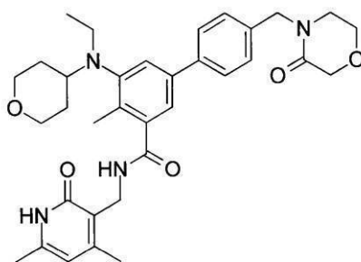
化合物131
