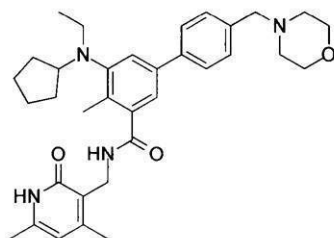
化合物36
