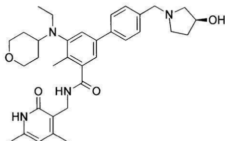
化合物70
