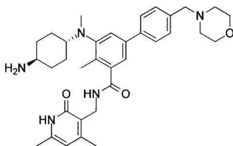
化合物43
