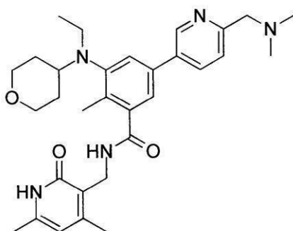
化合物110
