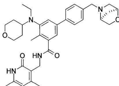
化合物68
