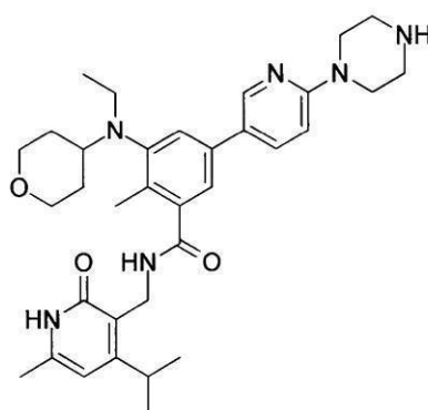
化合物185
