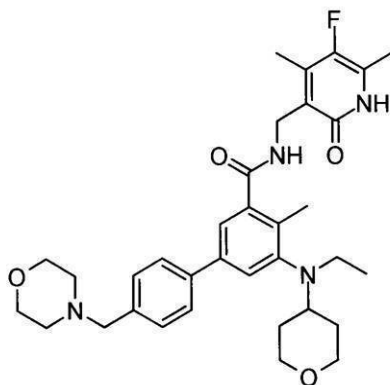
化合物179
