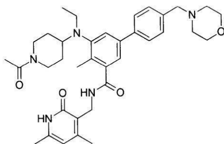
化合物125
