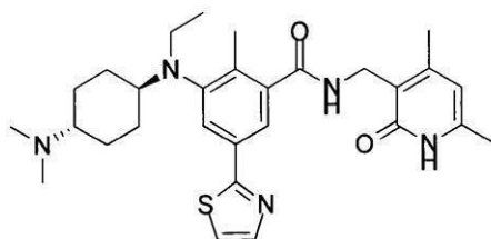
化合物168
