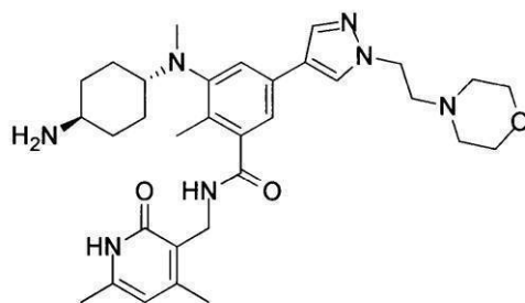
化合物51
