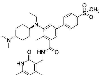
化合物150
