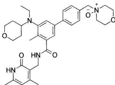
化合物137
