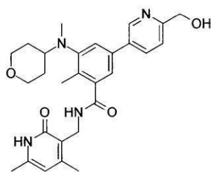
化合物29
