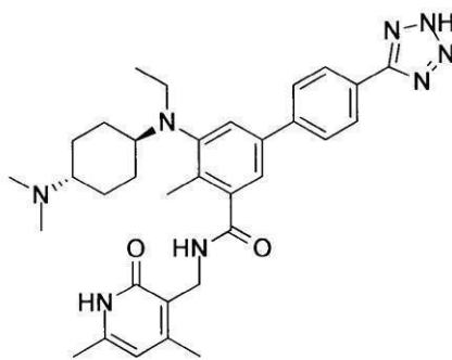
化合物163
