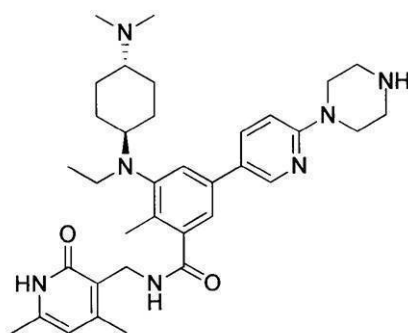
化合物172
