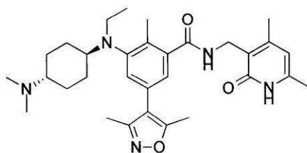
化合物159
