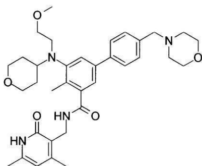
化合物142
