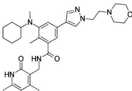
化合物15
