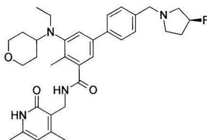
化合物72
