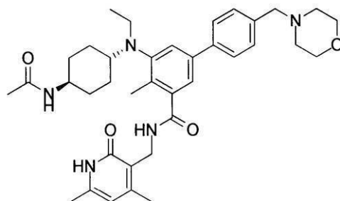
化合物129
