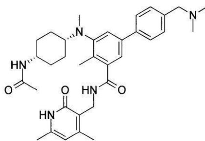
化合物40
