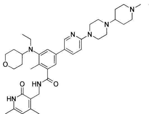
化合物187
