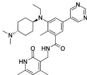
化合物151
