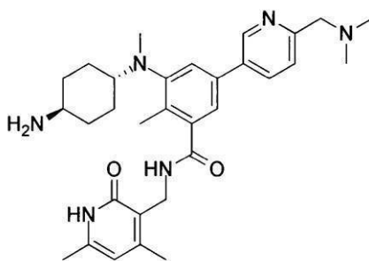
化合物53
