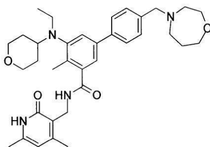
化合物88
