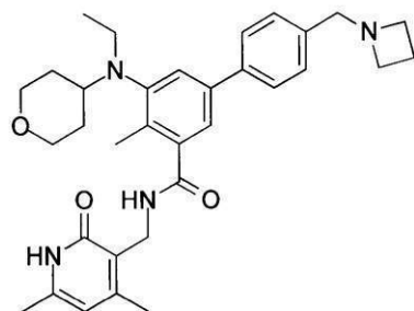
化合物82
