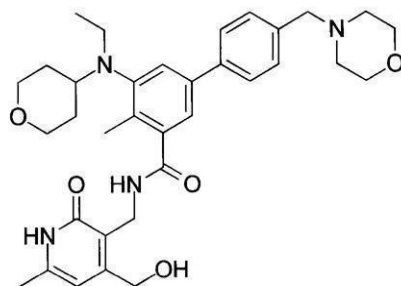
化合物118
