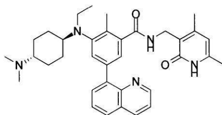
化合物153
