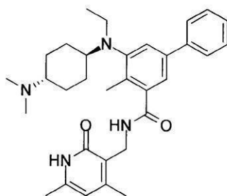
化合物147
