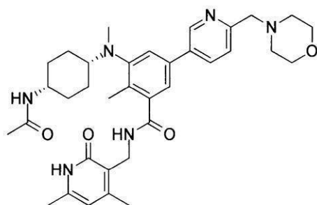
化合物57
