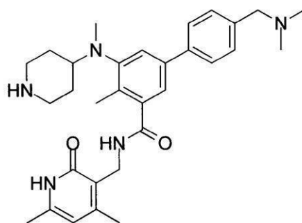
化合物27
