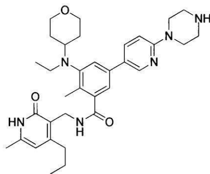
化合物184
