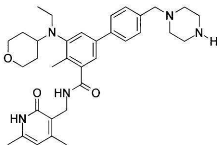
化合物73
