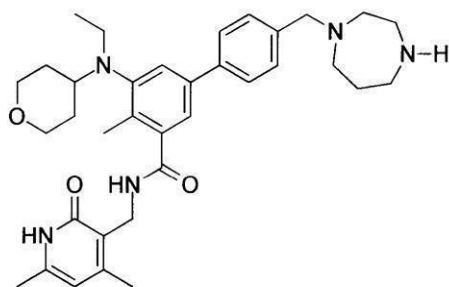
化合物86
