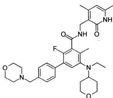
化合物130
