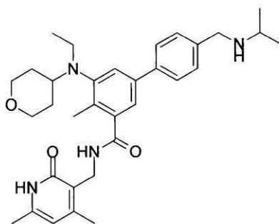
化合物92
