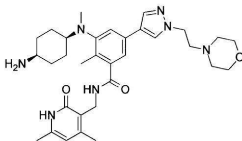
化合物48
