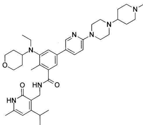
化合物188
