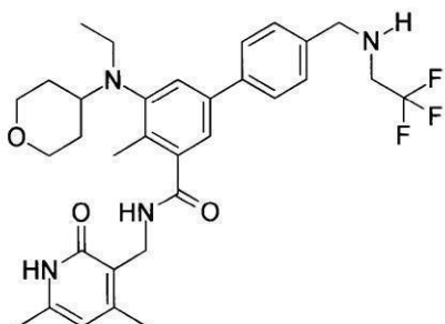
化合物104
