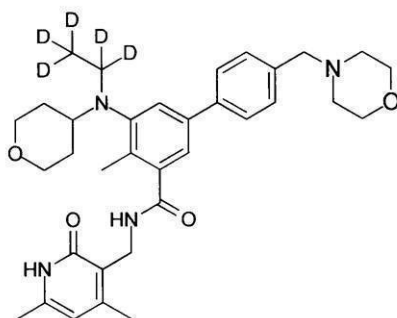
化合物143
