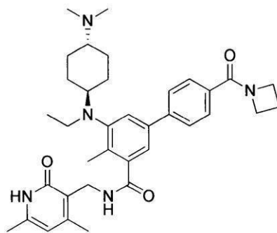
化合物181
