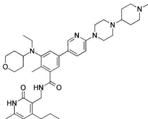
化合物189
