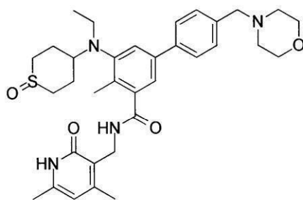
化合物133
