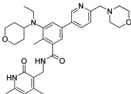
化合物64
