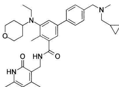
化合物97
