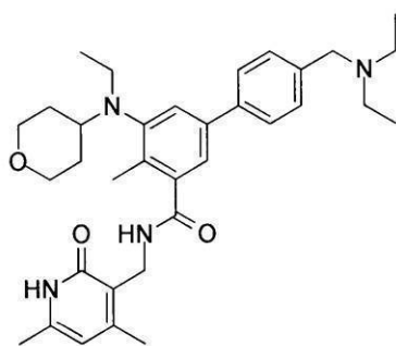
化合物94
