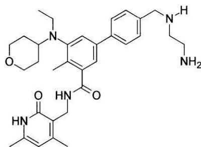
化合物101
