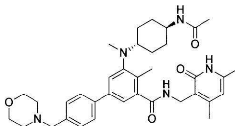
化合物21
