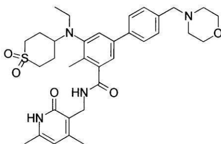
化合物136
