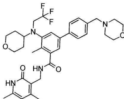
化合物138
