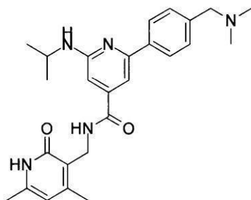
化合物 7
