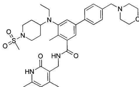
化合物124
