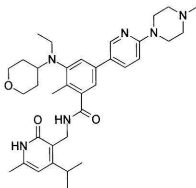
化合物186
