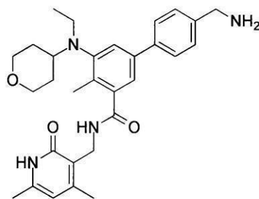
化合物89
