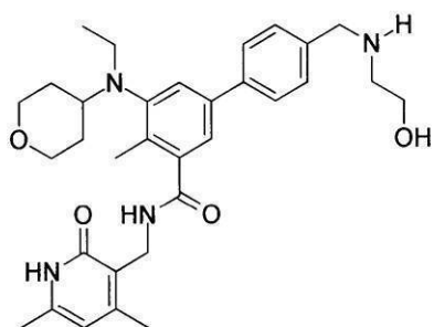
化合物98
