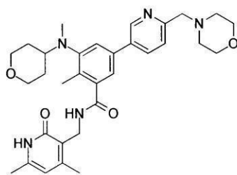
化合物28
