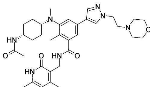
化合物38
