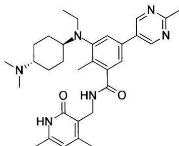
化合物164
