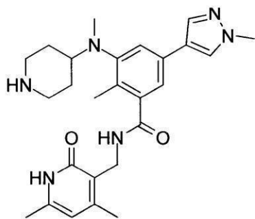
化合物26
