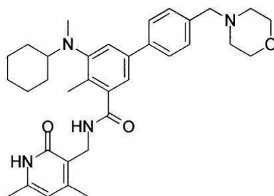
化合物14
