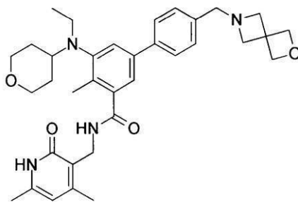
化合物105
