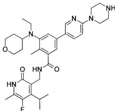
化合物195
