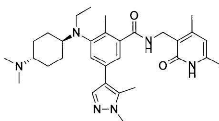
化合物160
