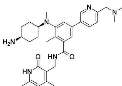
化合物52
