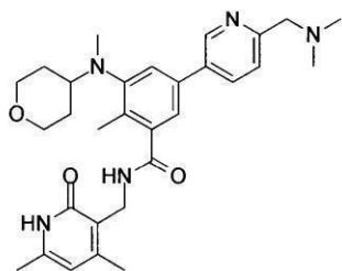
化合物30
