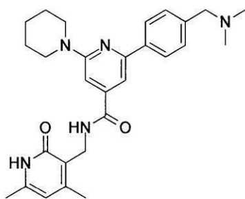
化合物6
