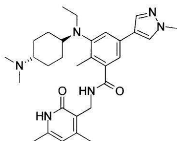
化合物145
