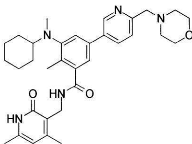
化合物31
