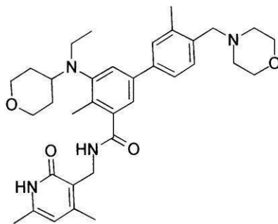
化合物134
