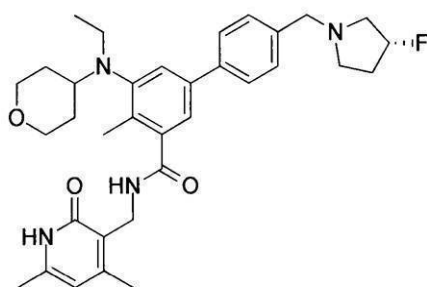
化合物74
