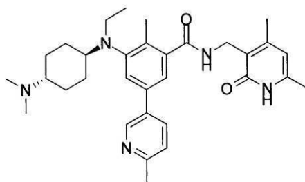
化合物158
