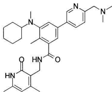
化合物32
