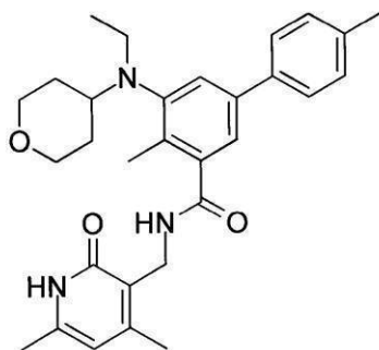
化合物112
