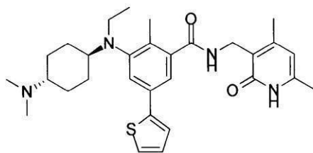
化合物167
