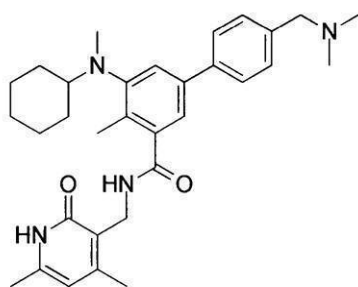
化合物16
