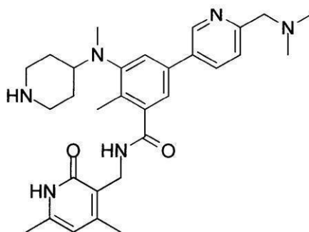
化合物41
