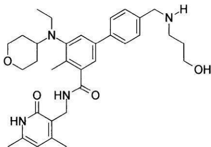
化合物99
