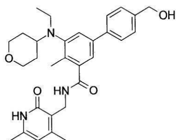
化合物113
