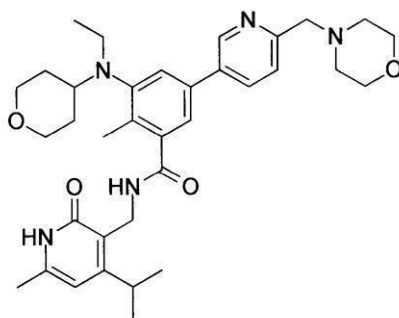
化合物190
