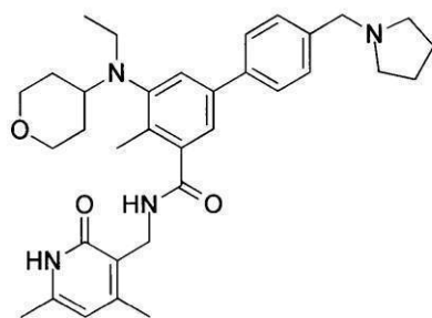
化合物69
