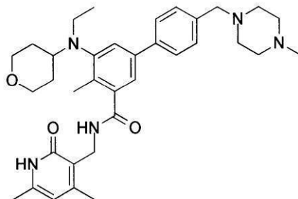
化合物66
