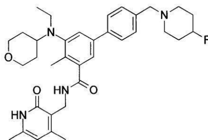
化合物80
