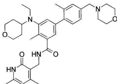
化合物122
