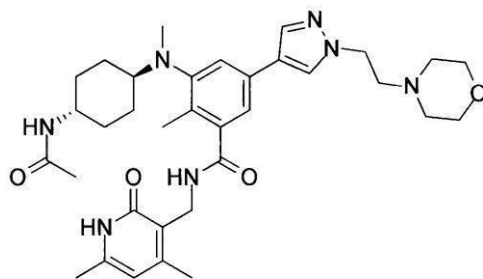
化合物37
