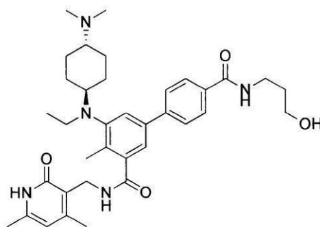
化合物182
