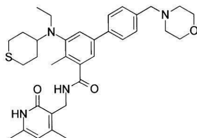
化合物132
