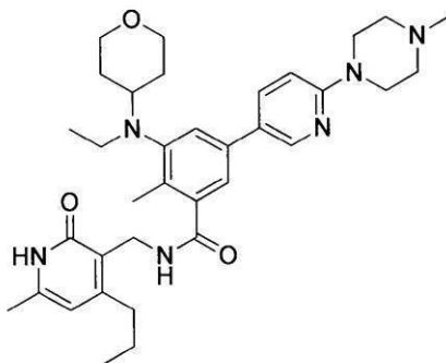
化合物183
