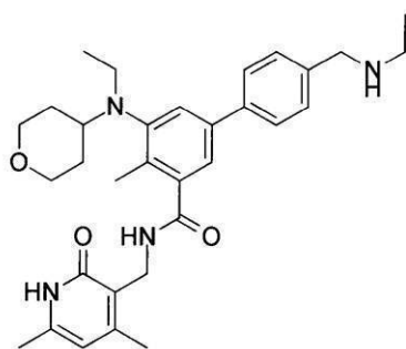
化合物91
