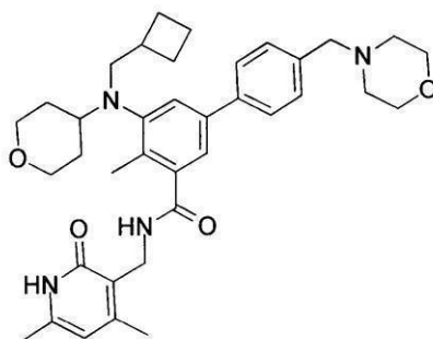
化合物63
