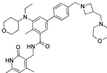
化合物115
