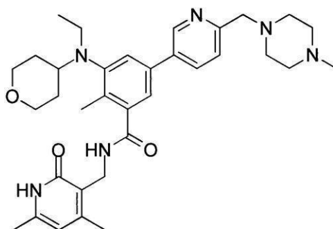
化合物111
