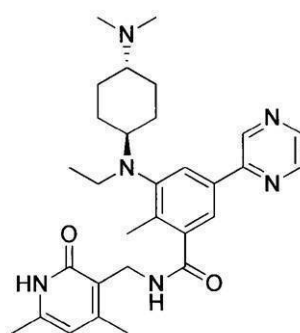
化合物174
