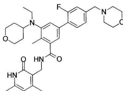
化合物121
