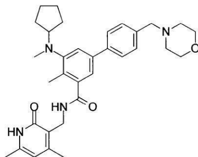
化合物2
