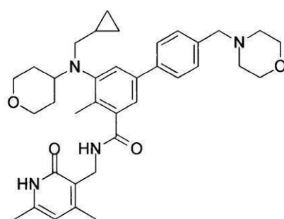
化合物61
