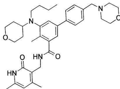
化合物62
