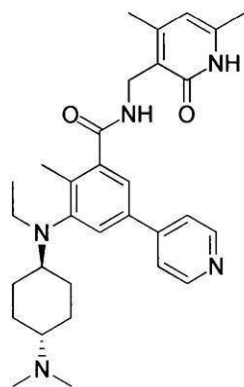
化合物155
