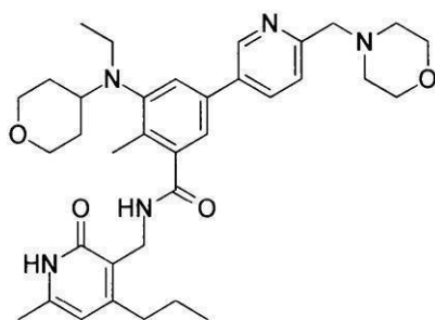
化合物191
