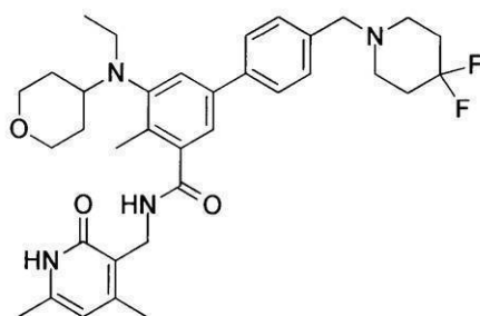
化合物81
