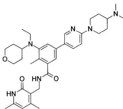
化合物192
