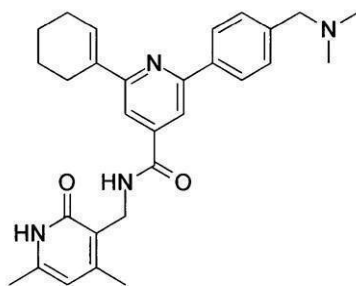
化合物5
