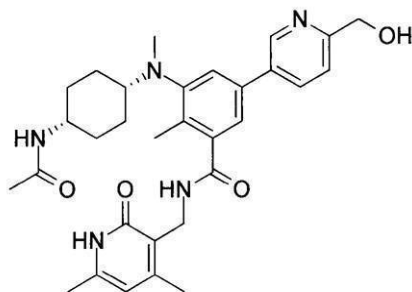
化合物56
