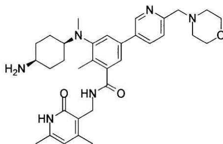
化合物49
