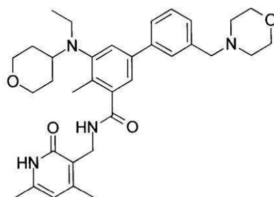
化合物114
