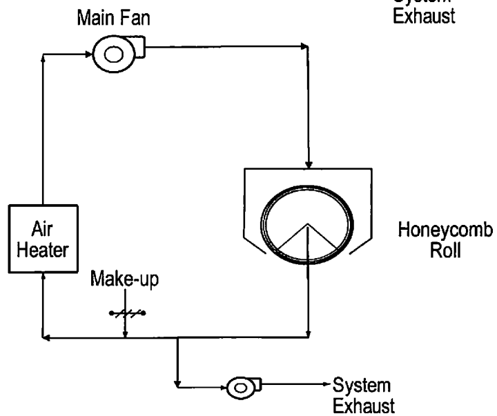
Valmet Schematic 3
