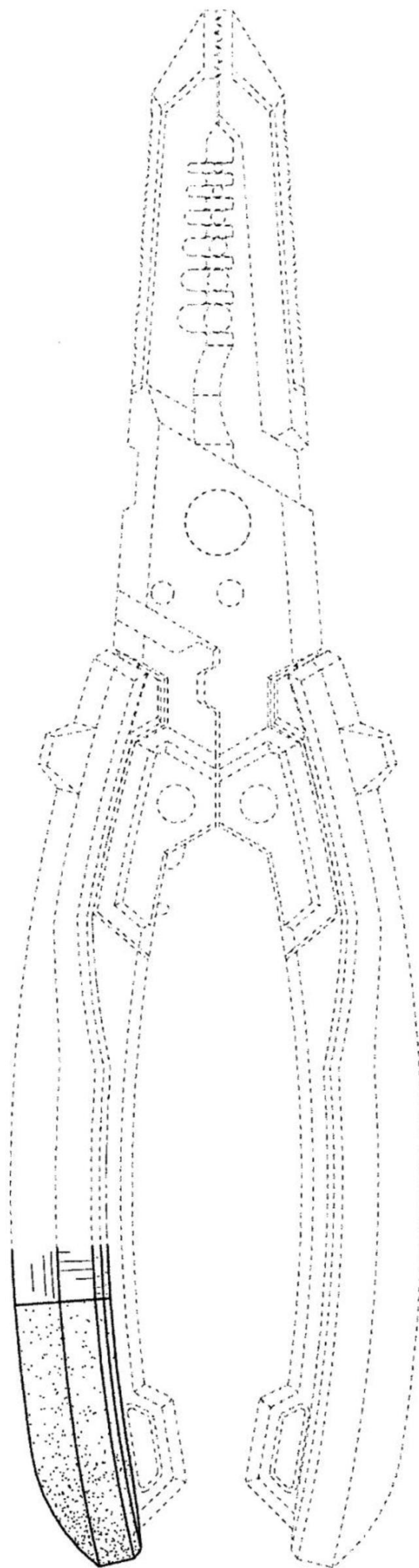
【前視圖】
