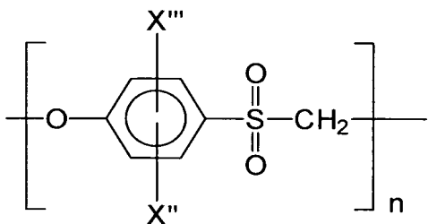
fórmula (IX)
