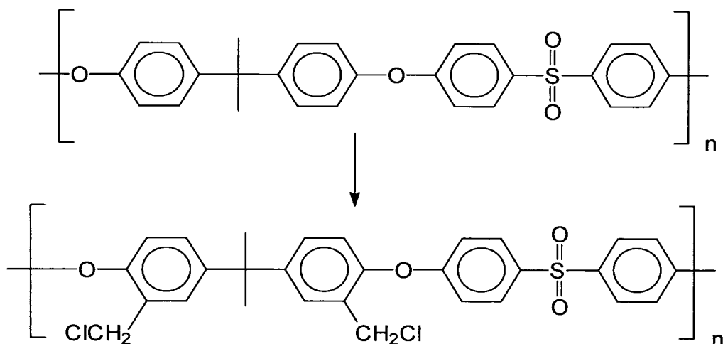
fórmula (IIA)
