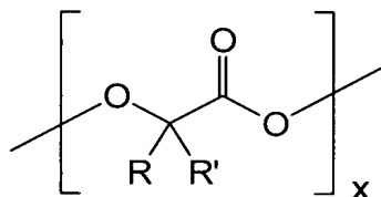
estrutura A
