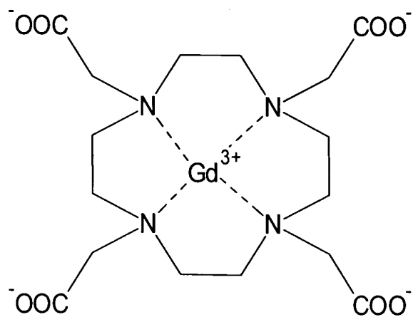
meglumina-gadoterato
