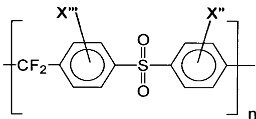
fórmula (VII)
