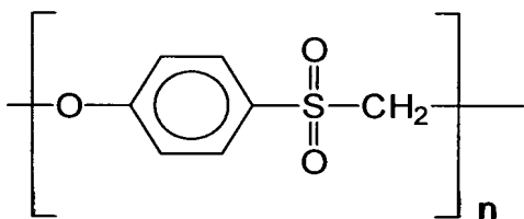
fórmula (V)
