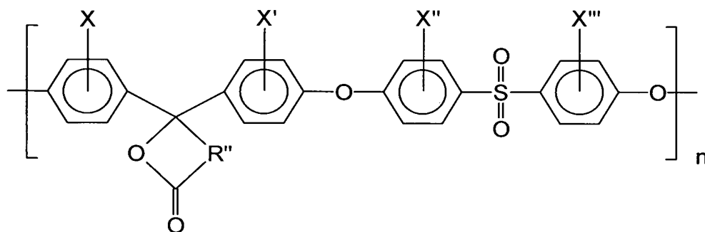
fórmula (XV)
