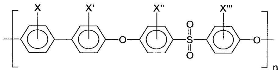
fórmula (XI)
