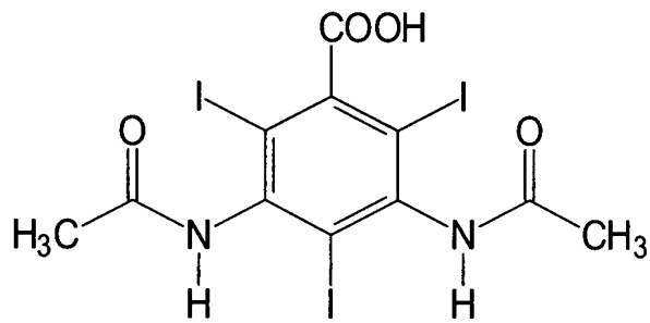
ácido amidotrizóico
