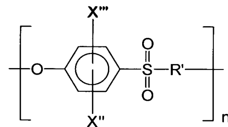
fórmula (VIII)
