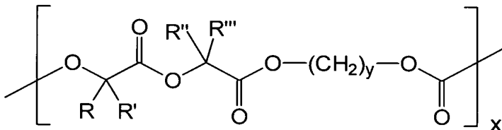
estrutura B
