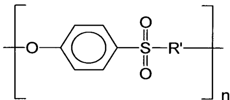
fórmula (III)
