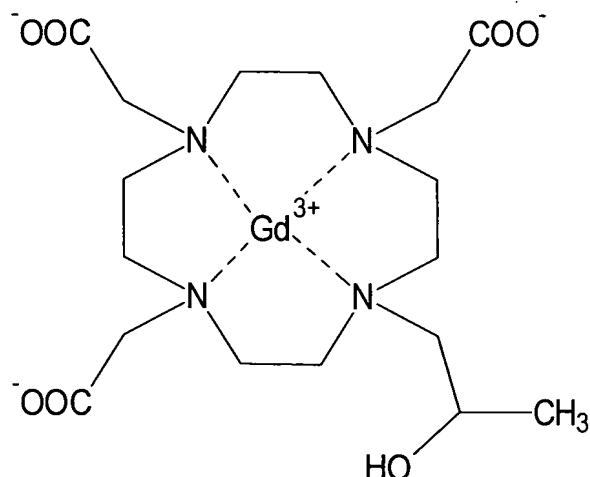
gadoteridol
