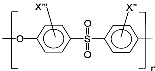
fórmula (IV)
