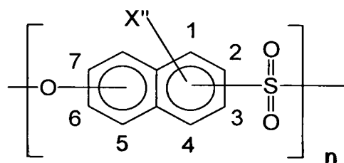
fórmula (VI)
