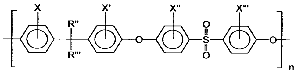
fórmula (XIII)
