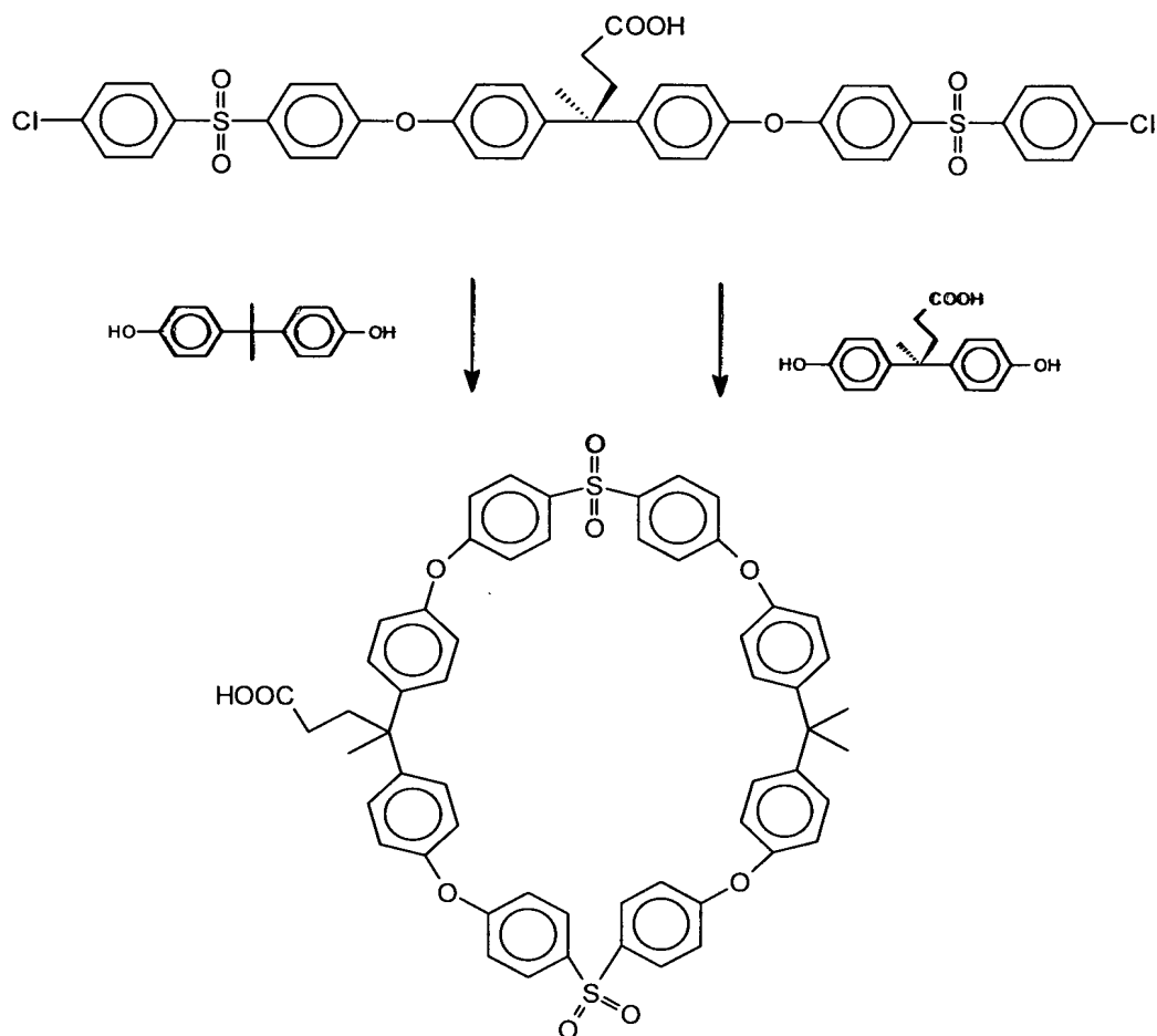
fórmula (XVI)
