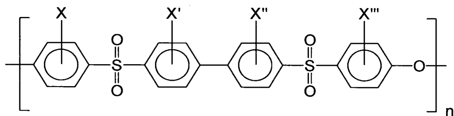
fórmula (XII)
