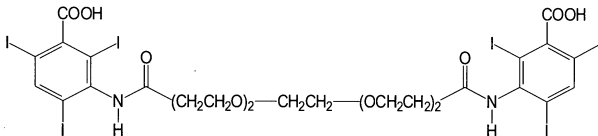
ácido iodoxamínico
