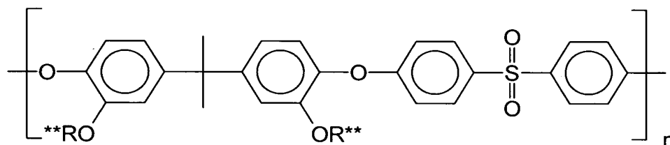
fórmula (IIB)
