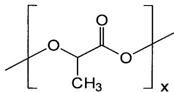
estrutura A1
