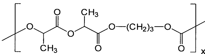
estrutura B1
