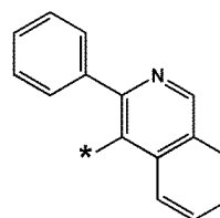
화학식 10-113
