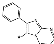
화학식 10-109
