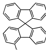
화학식 6-80
