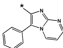
화학식 10-108
