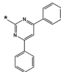
화학식 10-98
