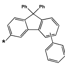
화학식 6-75
