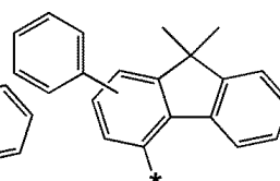
화학식 6-60
