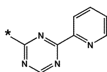
화학식 10-67
