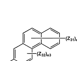
화학식 5-9
