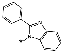
화학식 10-107
