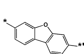
화학식 4-16
