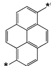
화학식 4-32
