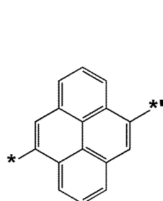
화학식 4-33
