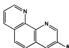
화학식 10-120
