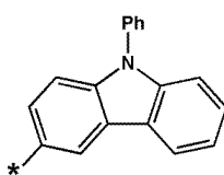
화학식 6-91
