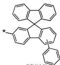
화학식 6-86
