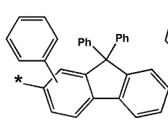
화학식 6-70
