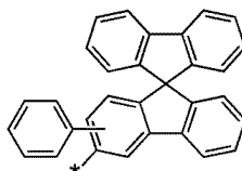
화학식 6-83
