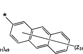
화학식 5-6
