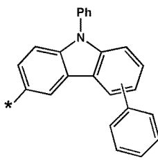
화학식 6-99
