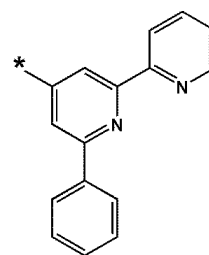
화학식 10-91
