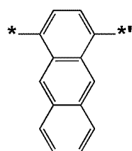
화학식 4-29
