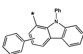
화학식 6-93
