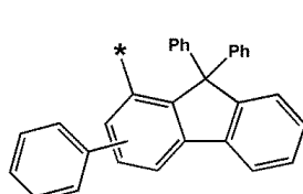
화학식 6-69
