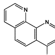
화학식 10-121
