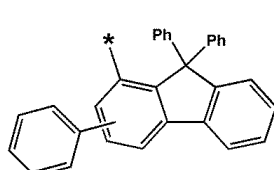
화학식 6-69
