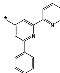
화학식 10-91
