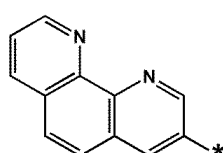
화학식 10-120
