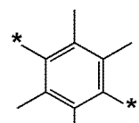
화학식 4-28
