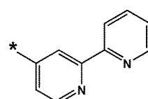
화학식 10-47
