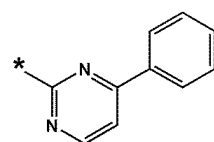
화학식 10-62
