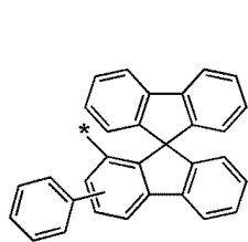
화학식 6-81
