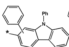
화학식 6-94
