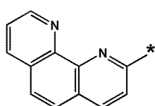
화학식 10-119
