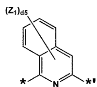
화학식 3-29
