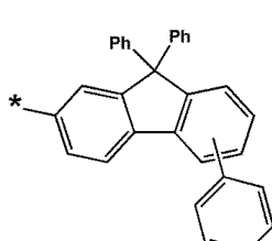
화학식 6-74
