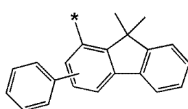
화학식 6-57
