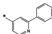
화학식 10-46
