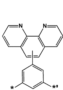
화학식 4-38
