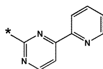
화학식 10-63
