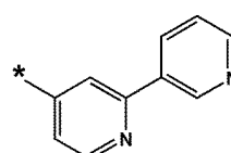
화학식 10-48
