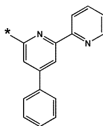
화학식 10-87
