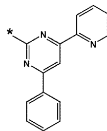
화학식 10-99
