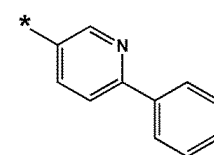
화학식 10-74
