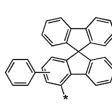
화학식 6-84
