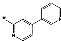
화학식 10-56
