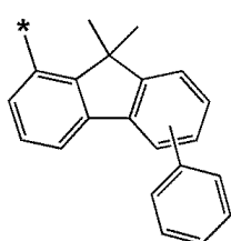
화학식 6-61
