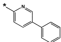
화학식 10-70
