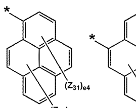
화학식 5-10
