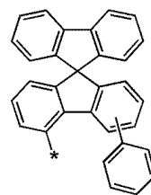
화학식 6-88
