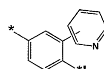
화학식 4-45
