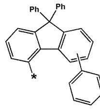
화학식 6-76
