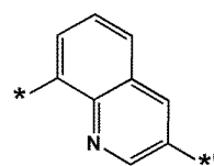
화학식 4-40
