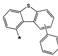
화학식 6-52
