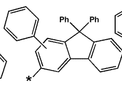
화학식 6-71
