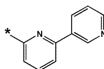
화학식 10-44
