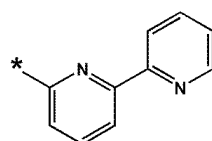
화학식 10-43
