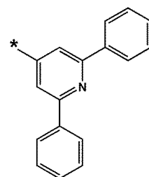
화학식 10-90
