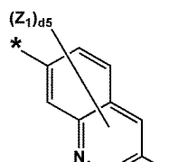
화학식 3-45
