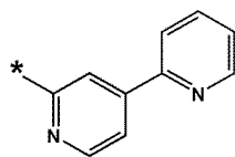
화학식 10-55
