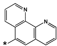
화학식 10-118
