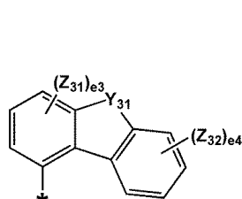
화학식 5-16
