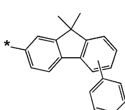
화학식 6-62
