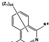
화학식 3-46
