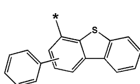
화학식 6-45
