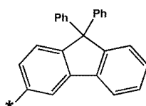
화학식 6-67
