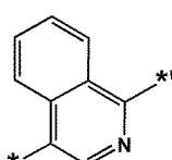
화학식 4-41
