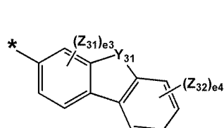
화학식 5-14
