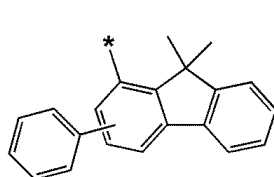
화학식 6-57
