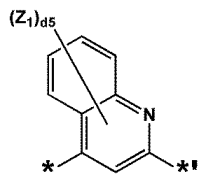
화학식 3-30
