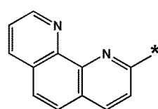
화학식 10-119
