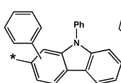
화학식 6-94
