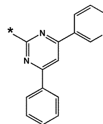
화학식 10-100
