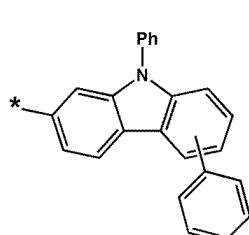
화학식 6-98
