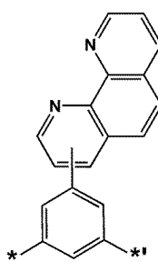
화학식 4-39
