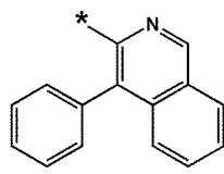
화학식 10-112
