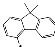
화학식 6-56
