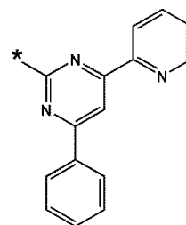
화학식 10-99
