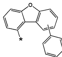
화학식 6-40
