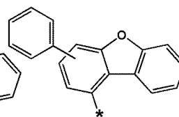
화학식 6-36
