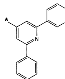
화학식 10-92
