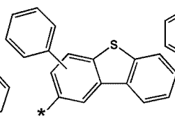
화학식 6-47
