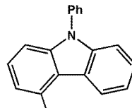
화학식 6-92
