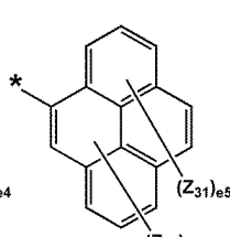
화학식 5-11
