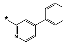
화학식 10-57
