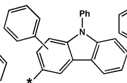
화학식 6-95
