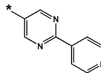
화학식 10-85
