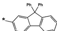
화학식 6-66
