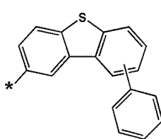
화학식 6-51
