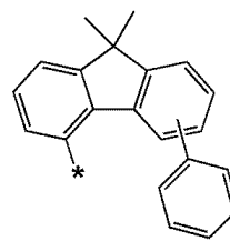
화학식 6-64
