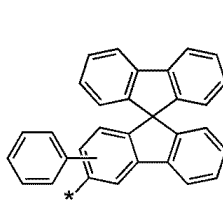
화학식 6-83
