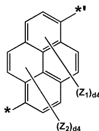
화학식 3-38
