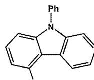
화학식 6-92
