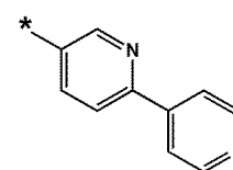
화학식 10-77
