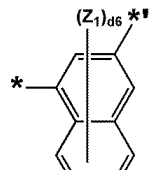
화학식 3-33
