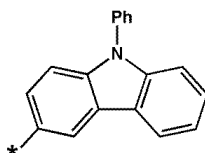
화학식 6-91
