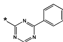
화학식 10-66
