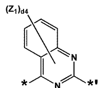
화학식 3-28
