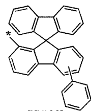
화학식 6-85
