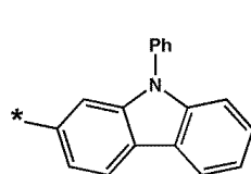
화학식 6-90
