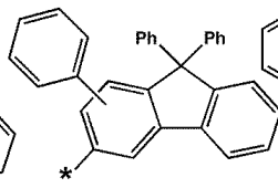
화학식 6-71
