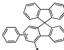
화학식 6-84
