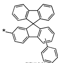
화학식 6-86
