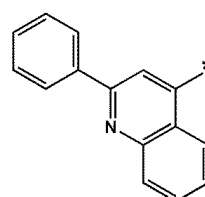
화학식 10-117
