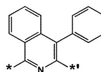
화학식 4-19
