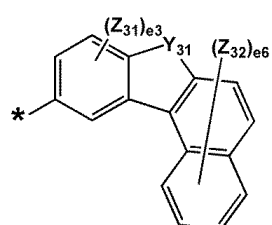
화학식 5-17
