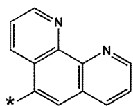
화학식 10-118
