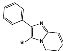
화학식 10-111
