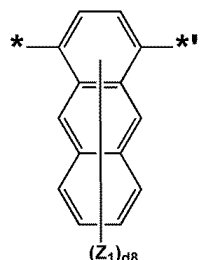
화학식 3-36
