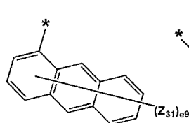
화학식 5-5
