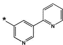
화학식 10-51
