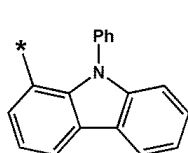
화학식 6-89
