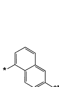
화학식 4-37
