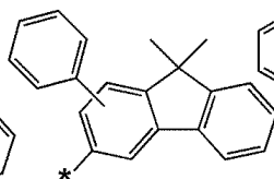
화학식 6-59
