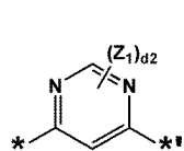
화학식 3-23
