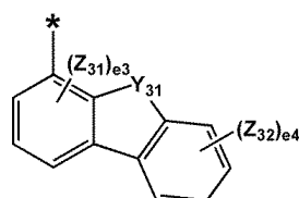
화학식 5-15
