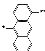
화학식 4-30
