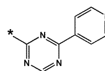
화학식 10-69
