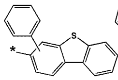
화학식 6-46
