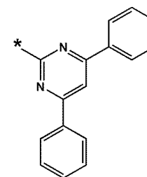
화학식 10-101
