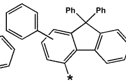
화학식 6-72
