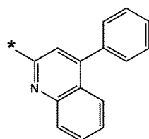
화학식 10-116
