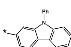
화학식 6-90
