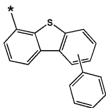
화학식 6-49
