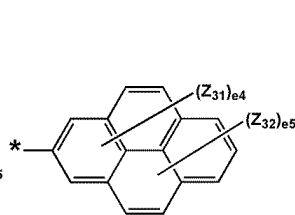
화학식 5-12
