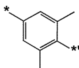
화학식 4-43
