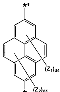
화학식 3-40
