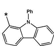
화학식 6-89
