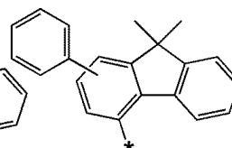
화학식 6-60
