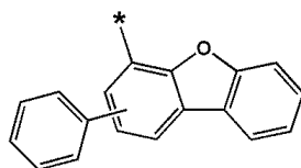
화학식 6-33
