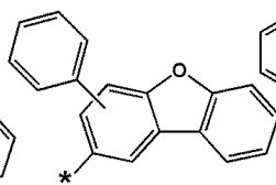
화학식 6-35
