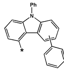
화학식 6-100
