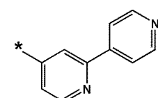
화학식 10-49
