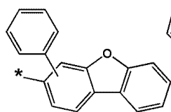
화학식 6-34
