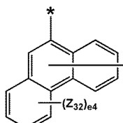
화학식 5-7
