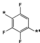
화학식 4-17
