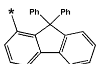
화학식 6-65
