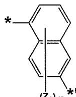
화학식 3-43
