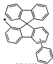
화학식 6-85
