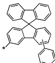
화학식 6-87
