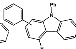
화학식 6-96
