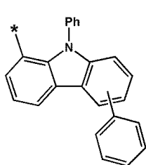
화학식 6-97
