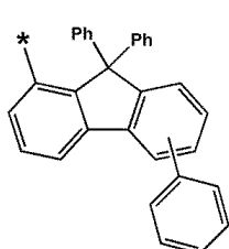
화학식 6-73
