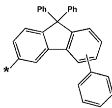
화학식 6-75
