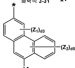
화학식 3-35
