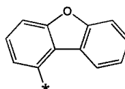
화학식 6-32
