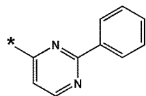
화학식 10-58
