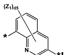
화학식 3-44
