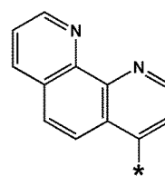
화학식 10-121
