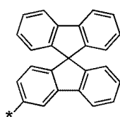
화학식 6-79
