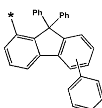
화학식 6-73
