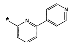
화학식 10-45
