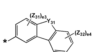
화학식 5-13
