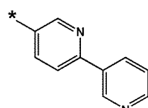
화학식 10-76
