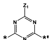
화학식 3-24
