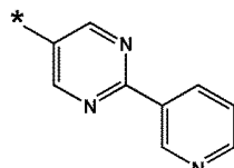
화학식 10-84
