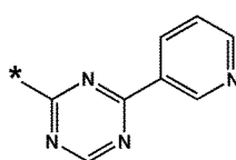
화학식 10-68
