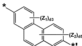
화학식 3-25
