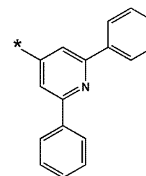
화학식 10-93
