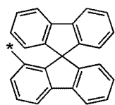
화학식 6-77
