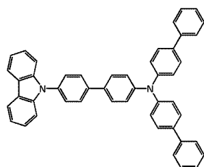
화합물 X
