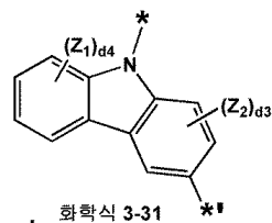
화학식 3-31
