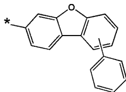
화학식 6-38
