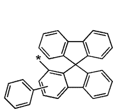
화학식 6-81
