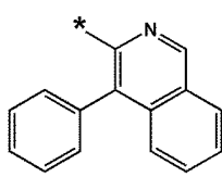
화학식 10-112
