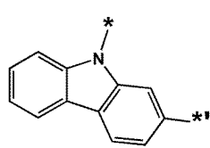
화학식 4-20
