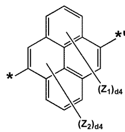
화학식 3-39
