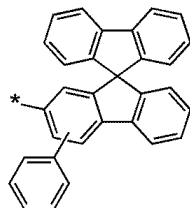
화학식 6-82
