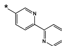
화학식 10-75
