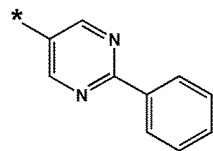
화학식 10-82
