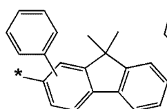
화학식 6-58
