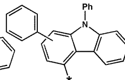
화학식 6-96
