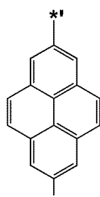
화학식 4-34
