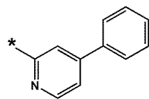
화학식 10-54
