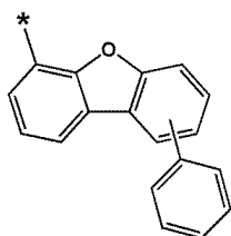
화학식 6-37
