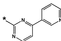
화학식 10-64
