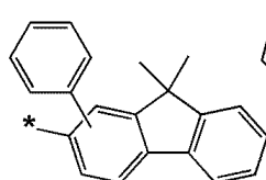
화학식 6-58
