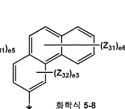
화학식 5-8
