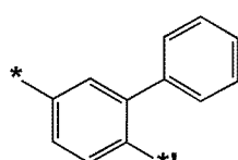
화학식 4-44
