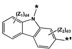
화학식 3-32
