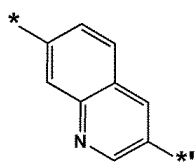
화학식 4-42
