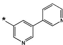
화학식 10-52
