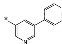
화학식 10-53
