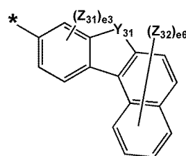
화학식 5-18
