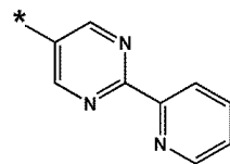
화학식 10-83
