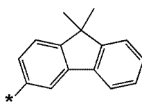
화학식 6-55
