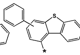
화학식 6-48
