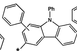
화학식 6-95
