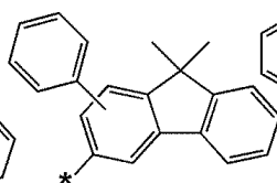
화학식 6-59
