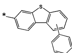
화학식 6-50
