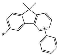
화학식 6-63
