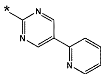
화학식 10-79
