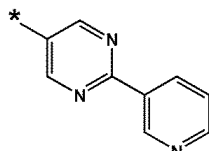
화학식 10-84
