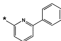
화학식 10-42
