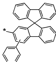
화학식 6-82
