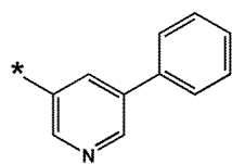
화학식 10-50
