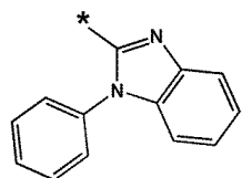
화학식 10-106
