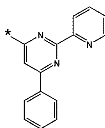
화학식 10-95
