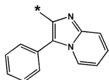
화학식 10-110
