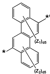
화학식 3-41
