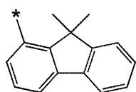
화학식 6-53
