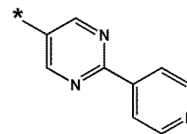
화학식 10-85
