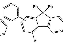
화학식 6-72
