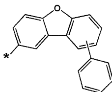
화학식 6-39
