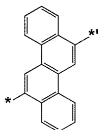
화학식 4-35
