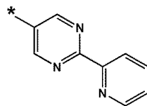
화학식 10-83
