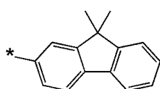
화학식 6-54
