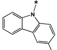
화학식 4-21
