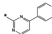
화학식 10-65
