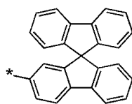
화학식 6-78
