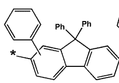
화학식 6-70
