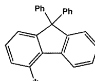
화학식 6-68
