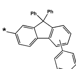
화학식 6-74
