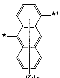
화학식 3-37
