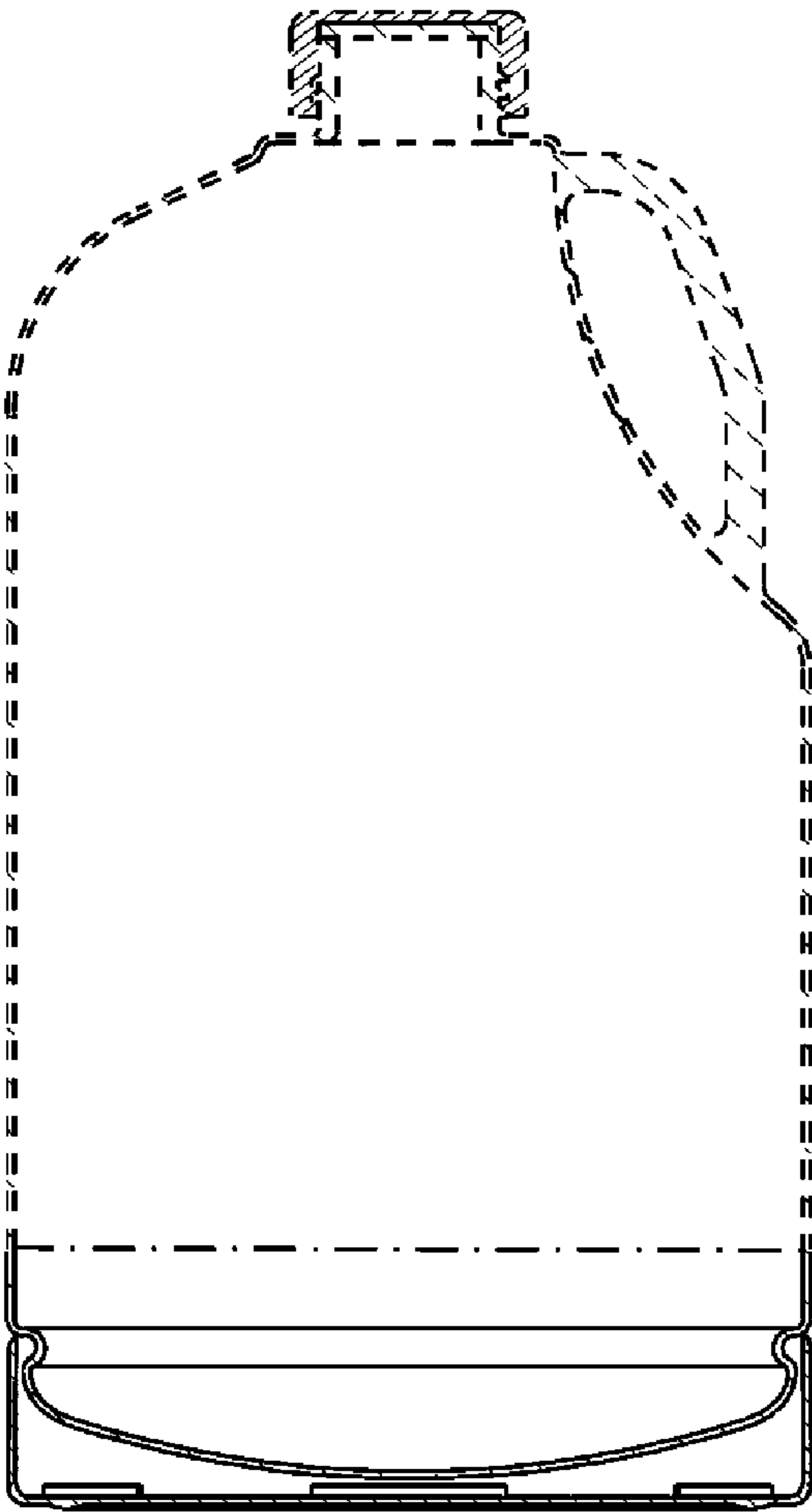
【A-A’ 剖面圖】
