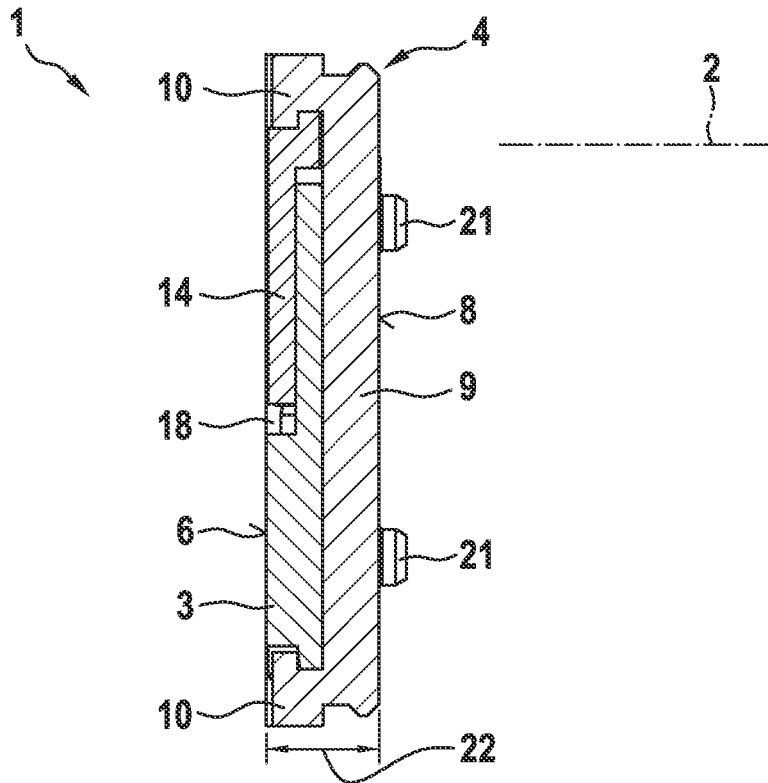
Fig. 5 A - A
