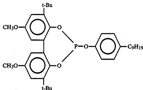
Ligand B
