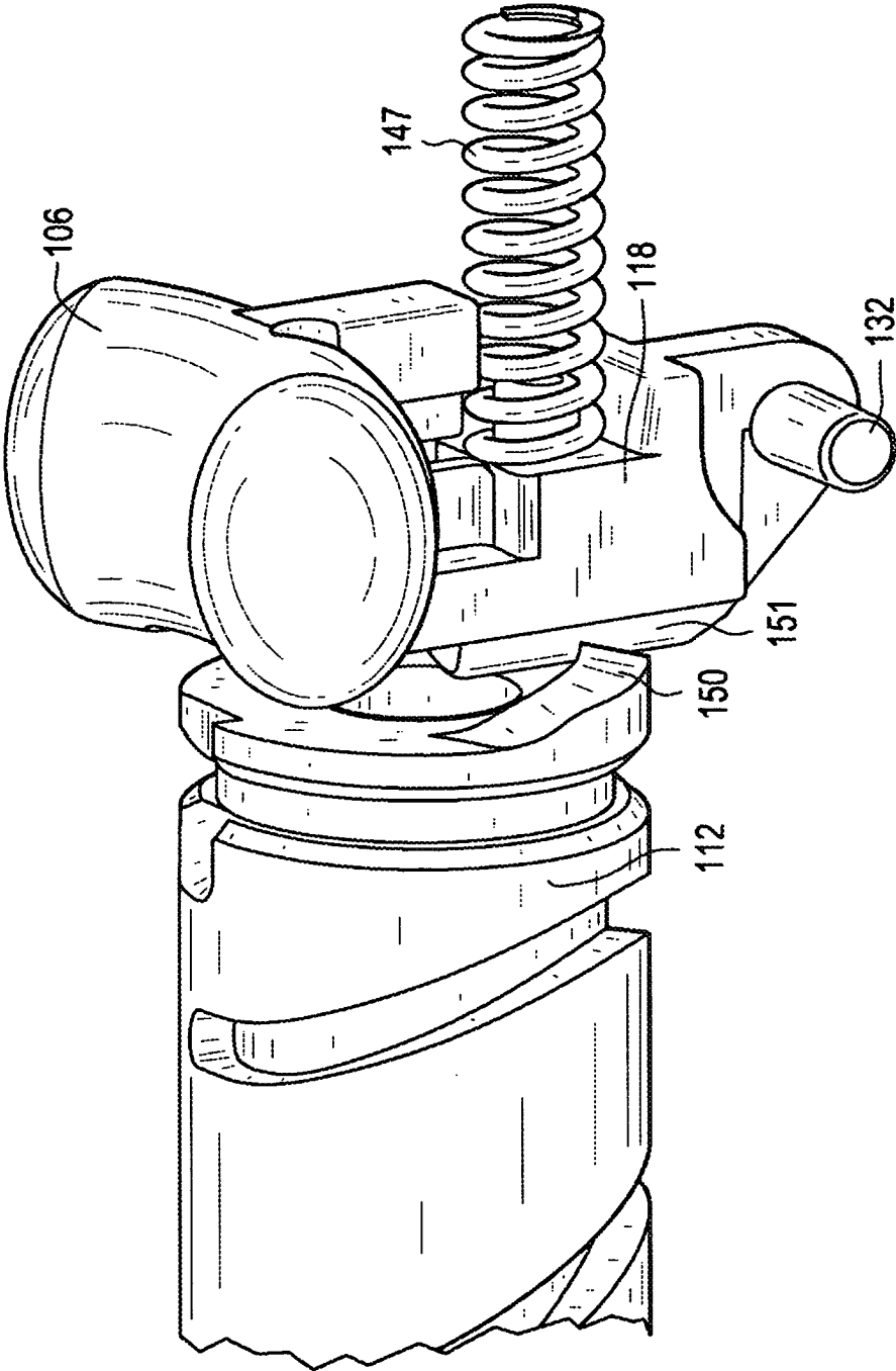
FIG. 1L
