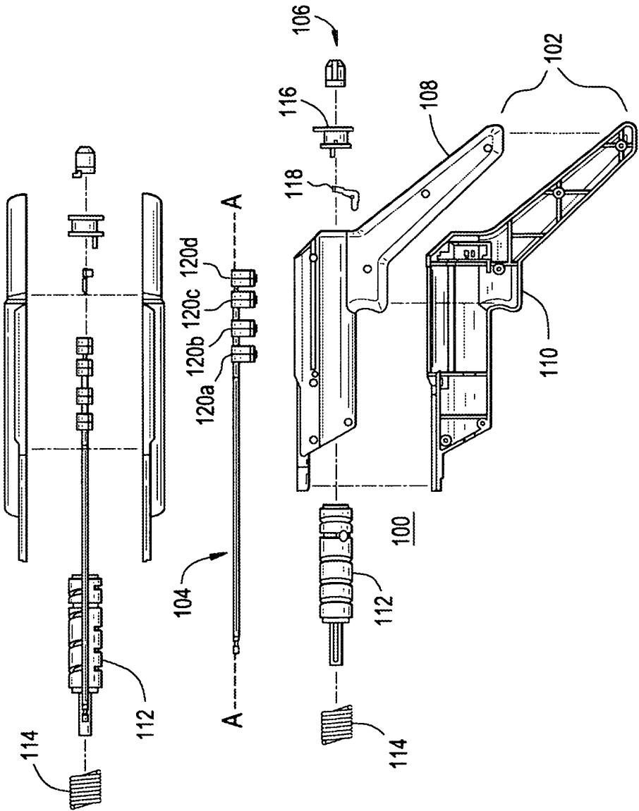
FIG. 1H
