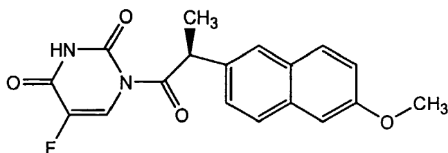
5FU-Naproxen (IV), and
