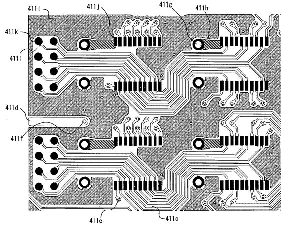
回路パターンの構成例の説明 1
