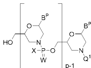
[B-1-1]
