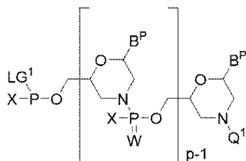
[B-1-2]
