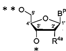
[4a1]
