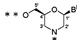
[4d1]
