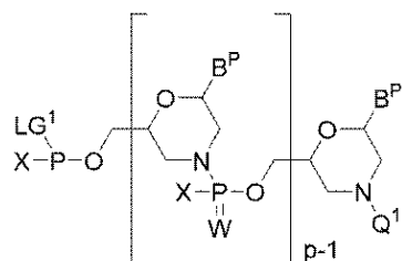
[B-1-2]
