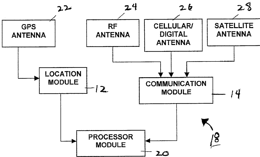
Fig. 9 The Antenna Module (D)
