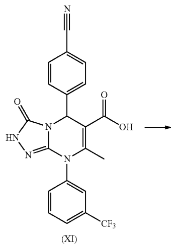
(XI)
