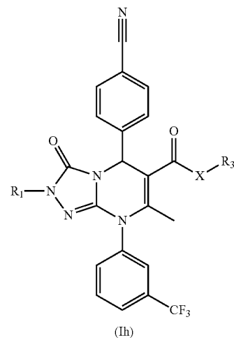
(Ih)
