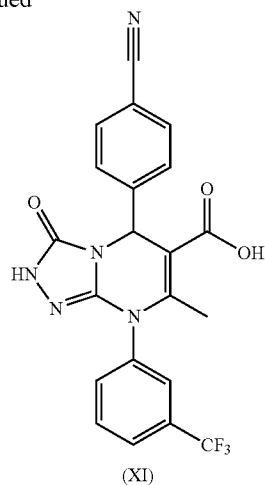
(XI)
