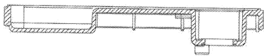
SECTION D-D
