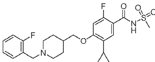
5-Cyclopropyl-2-fluoro-4-((1-(2-fluorobenzyl)piperidin-4-yl)methoxy)-N-(methylsulfonyl)benzamide
