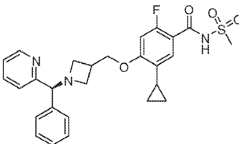
(S)-5-Cyclopropyl-2-fluoro-N-(methylsulfonyl)-4-((1-(phenyl(pyridin-2-yl)methyl)azetidin-3-yl)methoxy)benzamide
