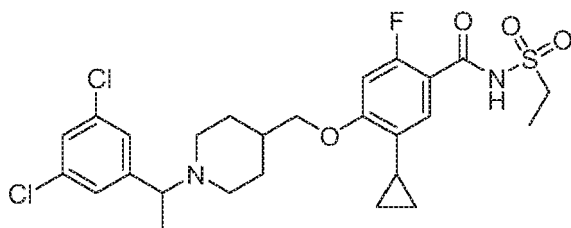
5-Cyclopropyl-4-((1-(1-(3,5-dichlorophenyl)ethyl)piperidin-4-yl)methoxy)-N-(ethylsulfonyl)-2-fluorobenzamide
