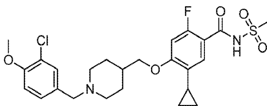
4-((1-(3-Chloro-4-methoxybenzyl)piperidin-4-yl)methoxy)-5-cyclopropyl-2-fluoro-N-(methylsulfonyl)benzamide
