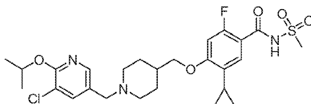
4-((1-((5-Chloro-6-isopropoxy)pyridin-3-yl)methyl)piperidin-4-yl)methoxy)-5-cyclopropyl-2-fluoro-N-(methylsulfonyl)benzamide
