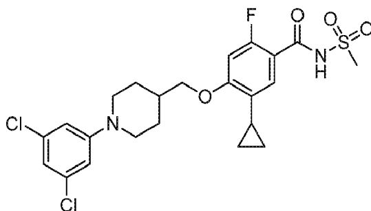
5-Cyclopropyl-4-((1-(3,5-dichlorophenyl)piperidin-4-yl)methoxy)-2-fluoro-N-(methylsulfonyl)benzamide
