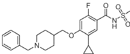
4-((1-Benzylpiperidin-4-yl)methoxy)-5-cyclopropyl-2-fluoro-N-(methylsulfonyl)benzamide
