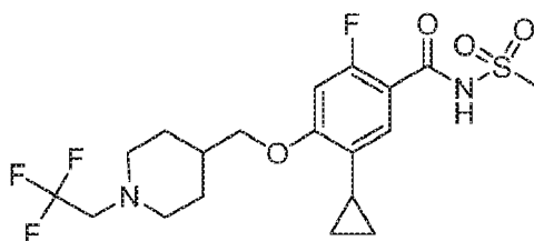
5-Cyclopropyl-2-fluoro-N-(methylsulfonyl)-4-((1-(2,2,2-trifluoroethyl)-piperidin-4-yl)methoxy)-benzamide
