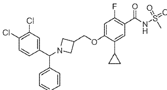
5-Cyclopropyl-4-((1-((3,4-dichlorophenyl)(phenyl)methyl)azetidin-3-yl)methoxy)-2-fluoro-N-(methylsulfonyl)benzamide
