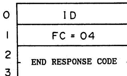
FIG. 4 E (END RESPONSE)
