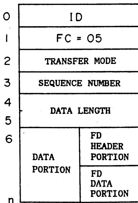
FIG. 4 F (NORMAL DATA)
