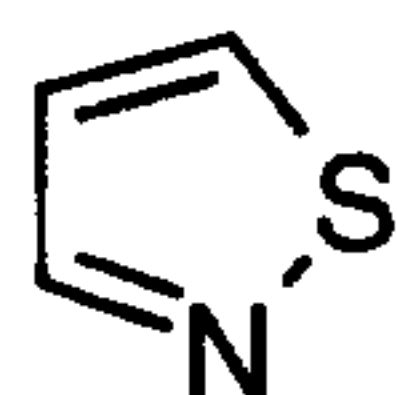
isothiazole (isothiazolyl)
