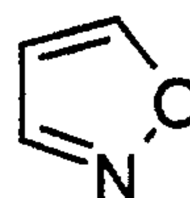
isoxazole (isoxazolyl)
