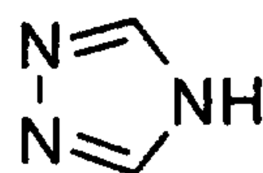
triazole (triazolyl)
