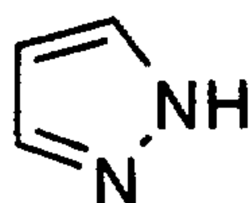
pyrazole (pyrazolyl)
