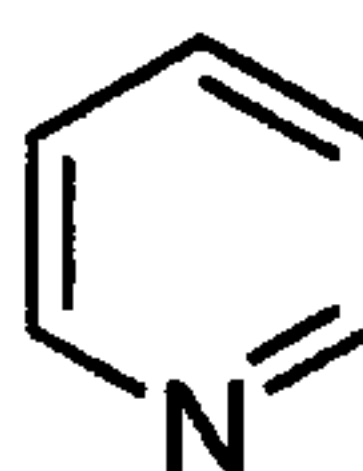
pyridine (pyridinyl)
