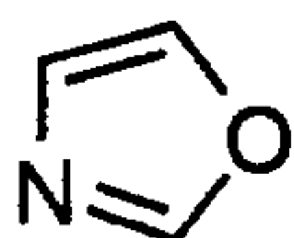
oxazole (oxazolyl)
