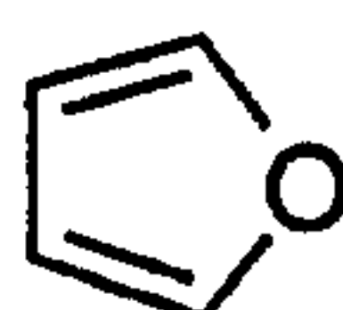
furan (furyl)
