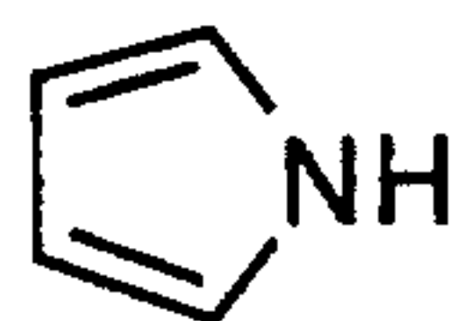
pyrrole (pyrrolyl)
