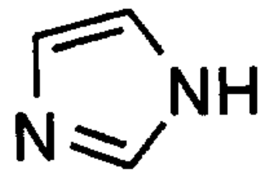
imidazole (imidazolyl)
