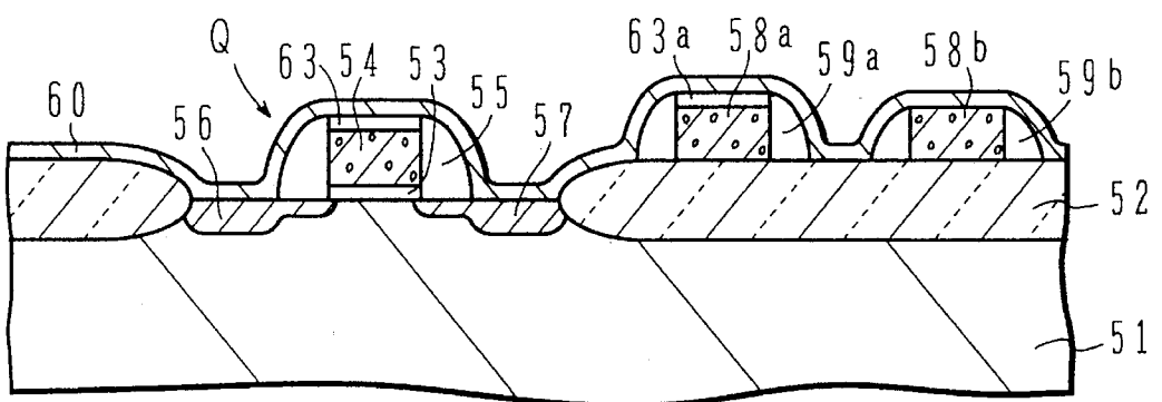
FIG. 14D
