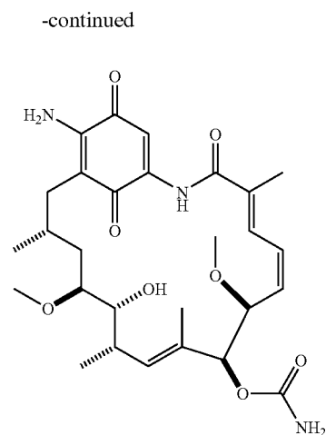
11-oxo-17-aminogeldanamycin
