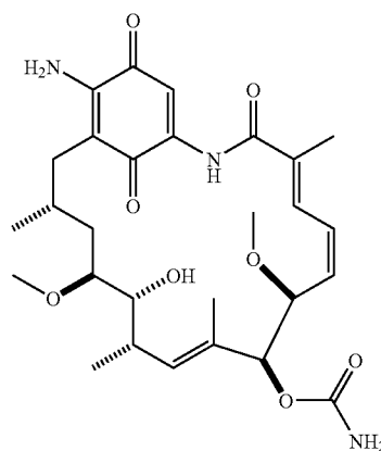
17-aminogeldanamycin
