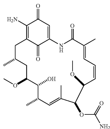
17-aminogeldanamycin
