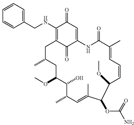
17-benzylaminogeldanamycin
