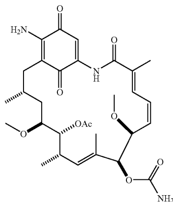
11-acetyl-17-aminogeldanamycin
