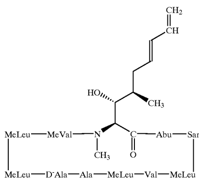
E-isomer
