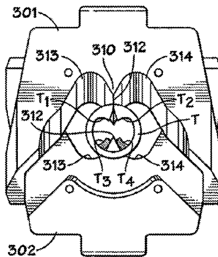
FIG. 15E
