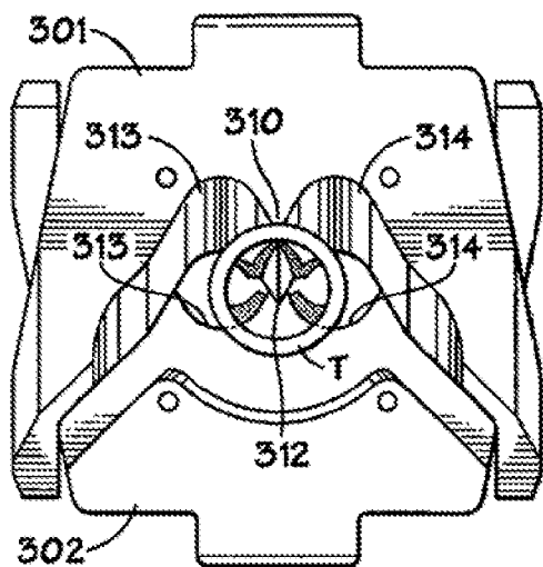
FIG. 15F
