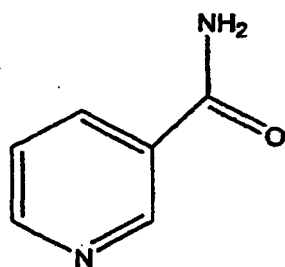
Nicotinamide (NA)
