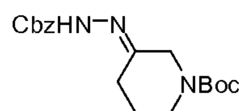
XV-Boc
