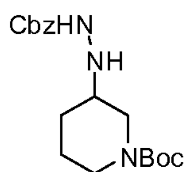
XVI-Boc
