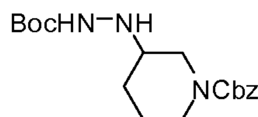
XVI-Cbz
