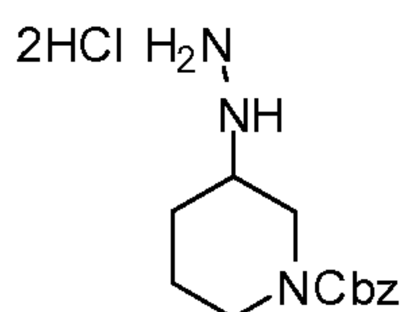
X-Cbz
