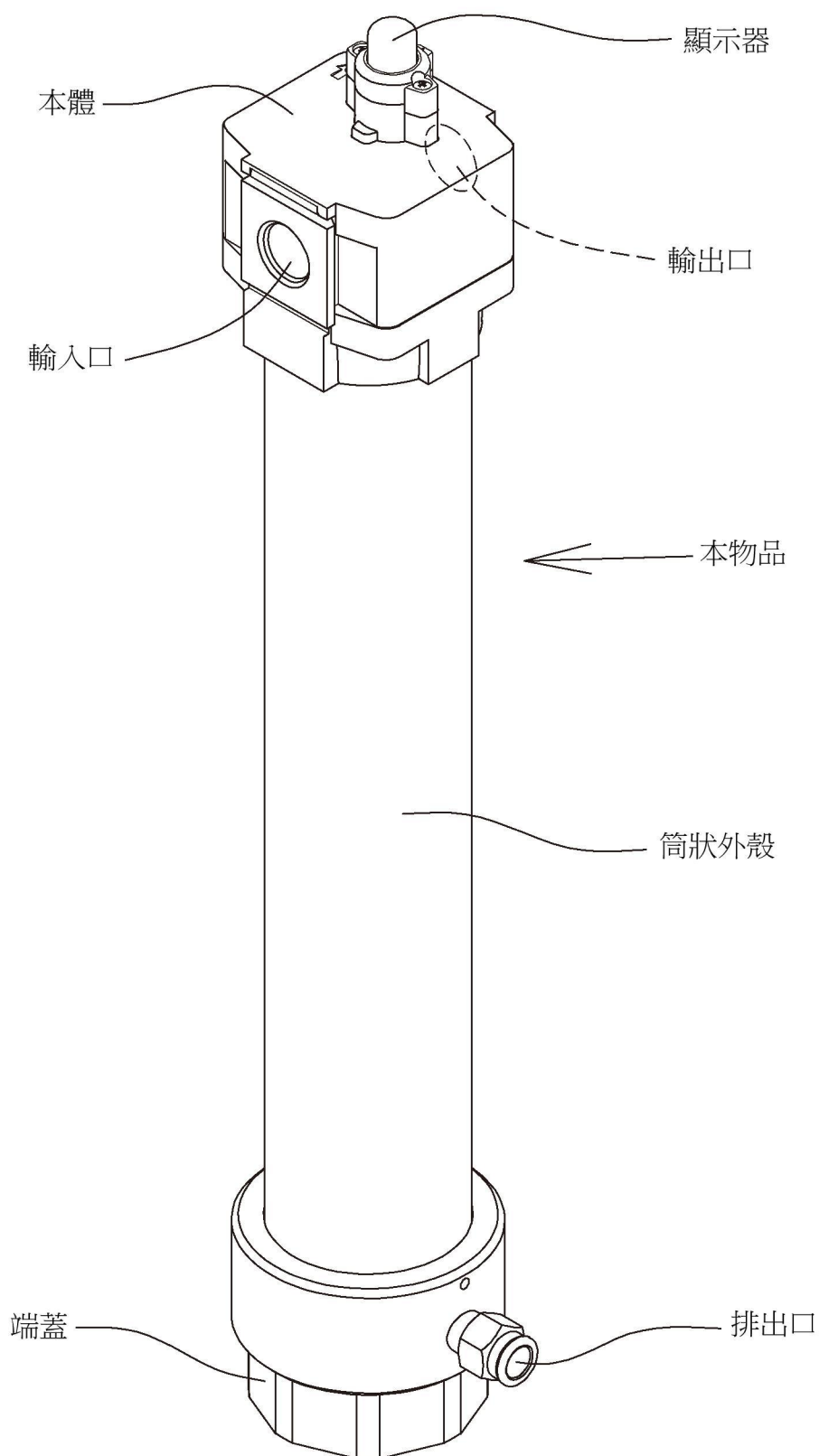
【參考圖】
