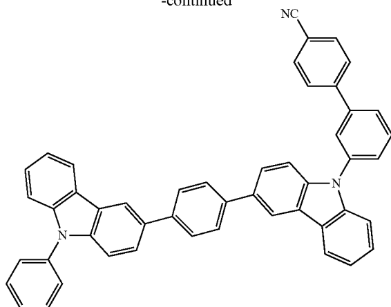
H11
