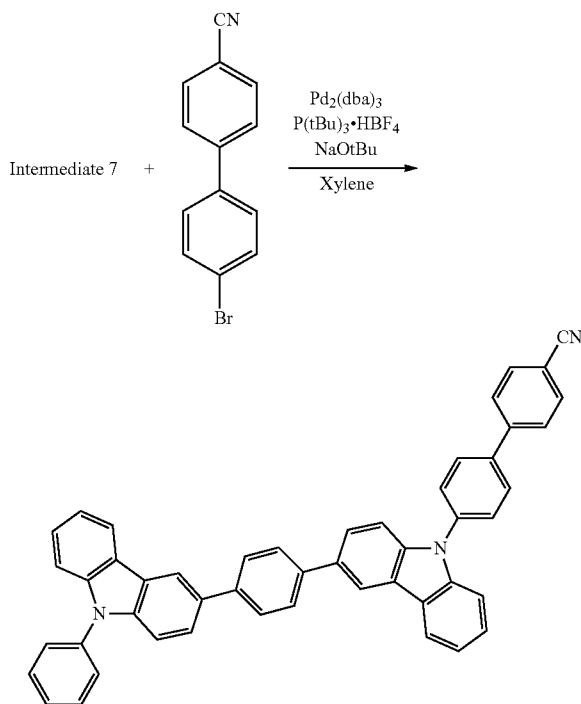
H10
