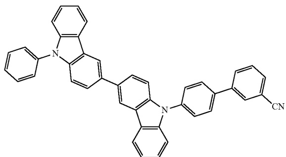
Compound F1
