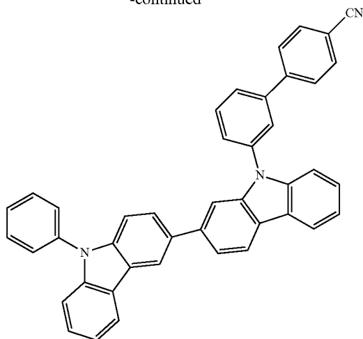
H4
