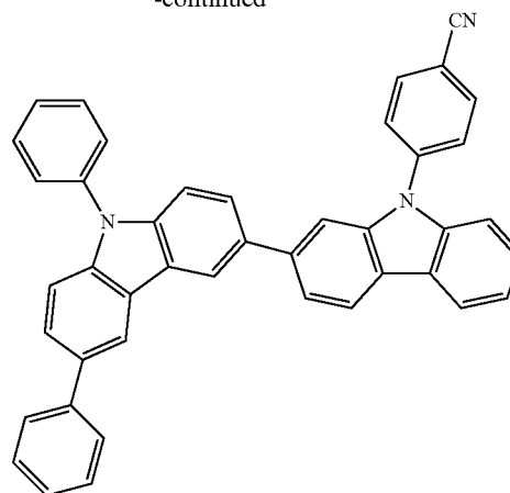
H16
