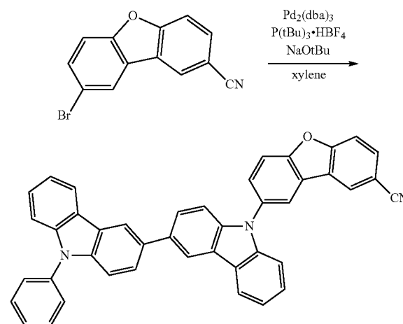
H13
