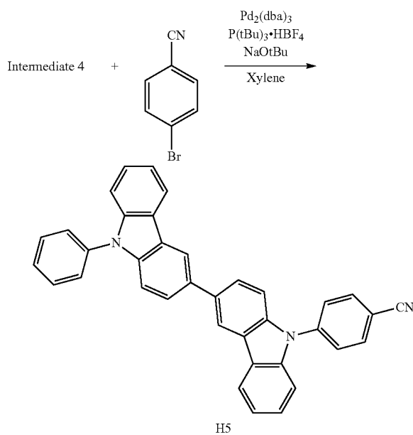
H5
