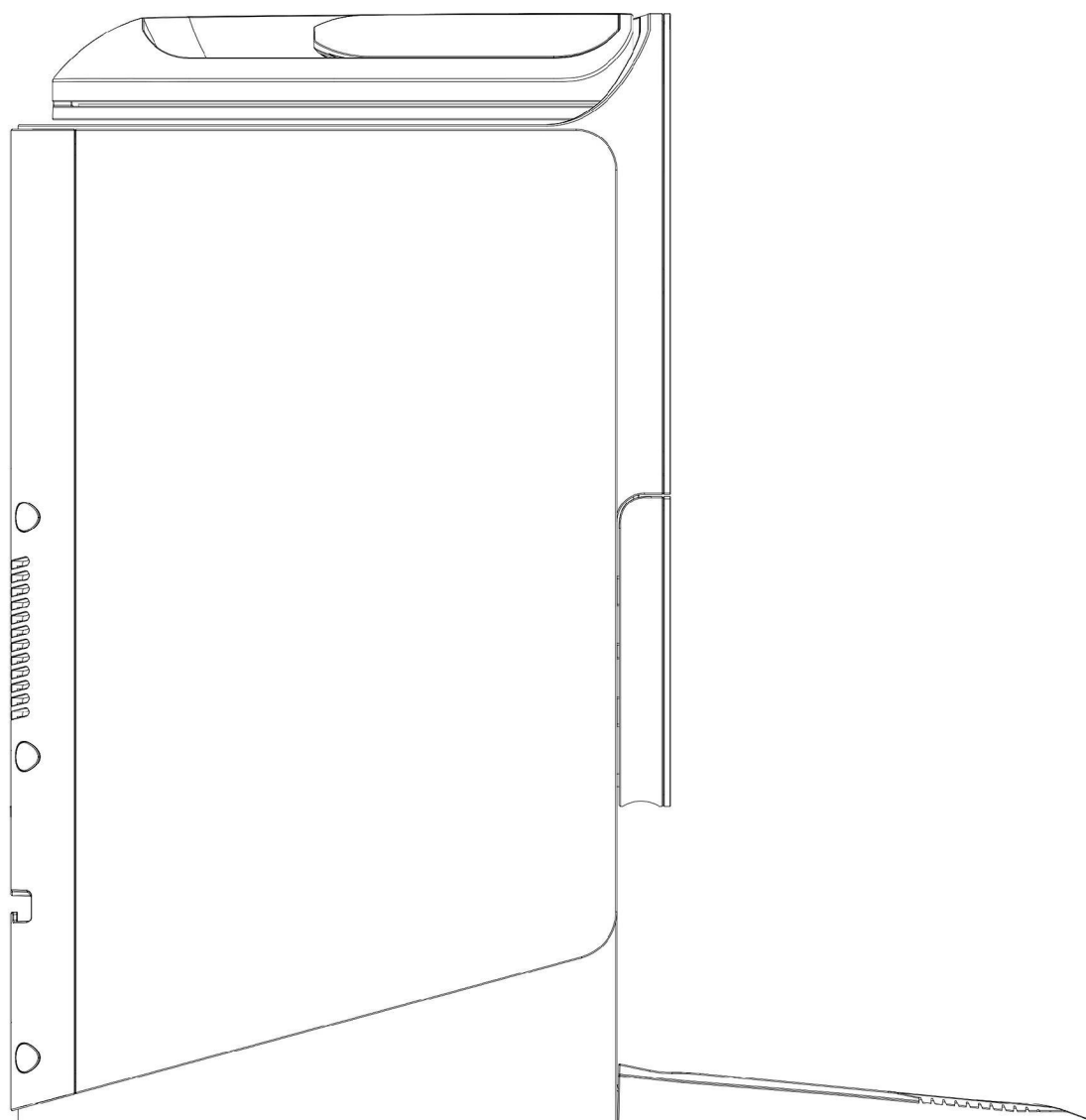
左側視圖
