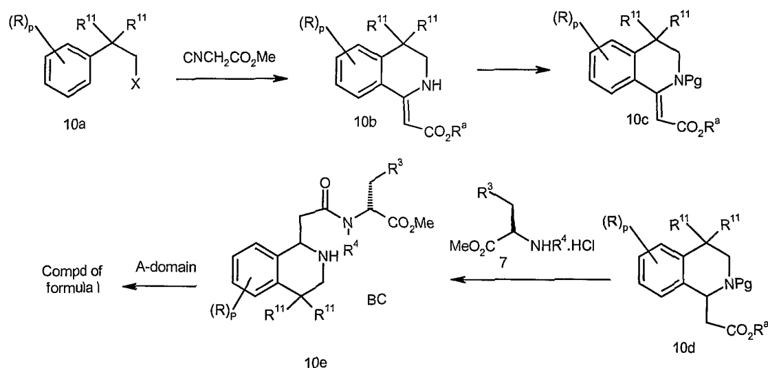
Scheme 10a
