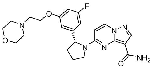
(R)-5-(2-(3-fluoro-5-(2-morpholinoethoxy)phenyl)pyrrolidin-1-yl)pyrazolo[1,5-a]pyrimidine-3-carboxamide
